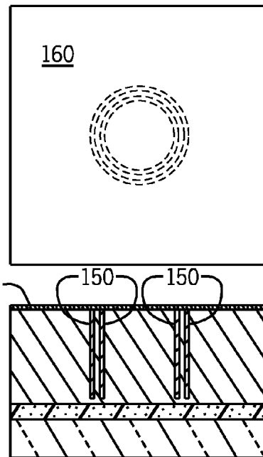
FIG. 14D
