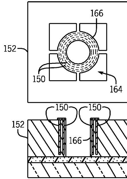
FIG. 14F
