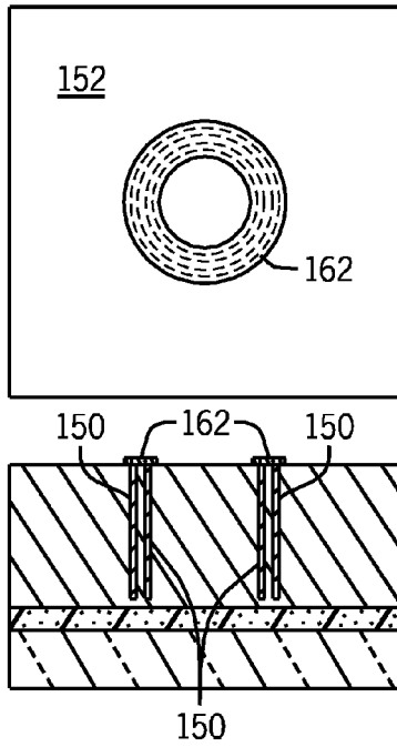
FIG. 14E
