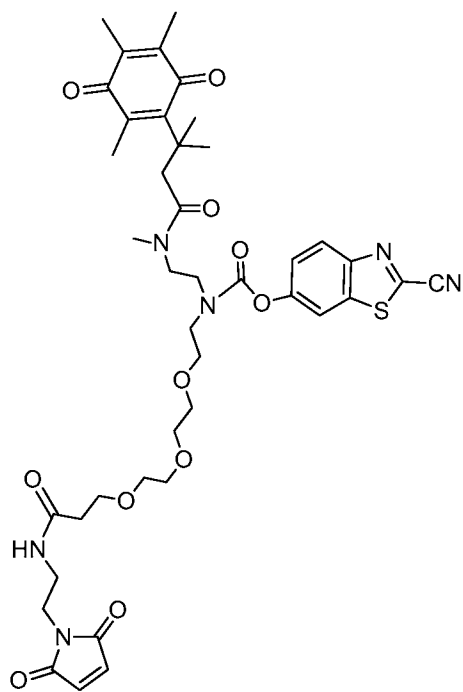
PBI 5916
