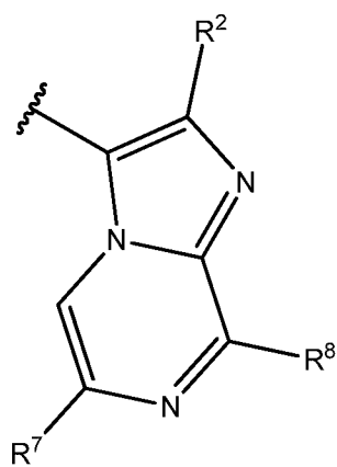
a coelenterazine ;
