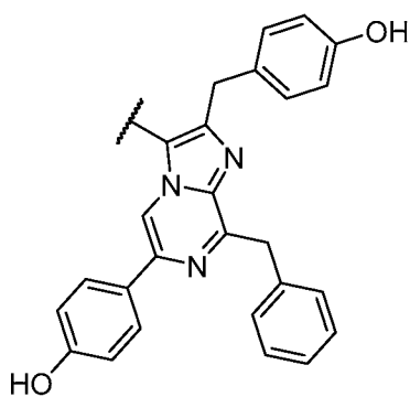
coelenterazine ;
