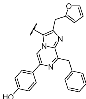
Furimazine H ;
