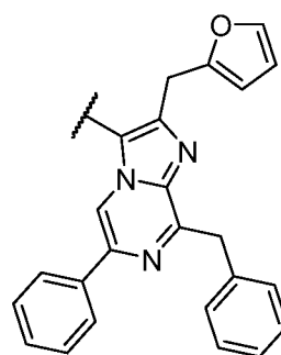
Furimazine ;
