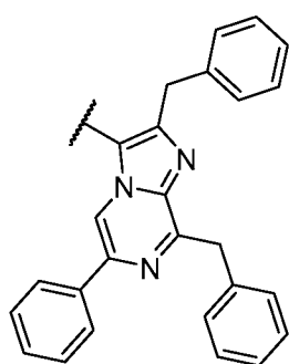
coelenterazine HH ;
