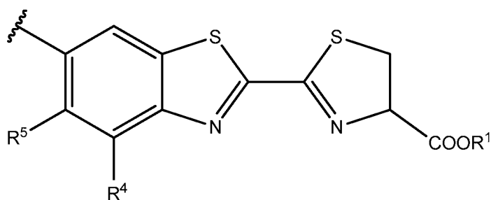
a luciferin ;
