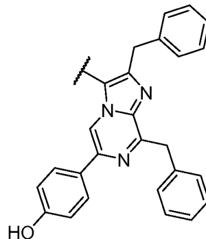
coelenterazine H ;
