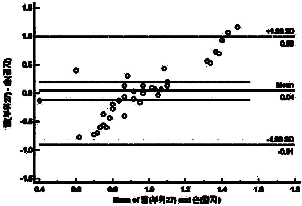
(c) 검지 손가락과 27부위의 RRI
