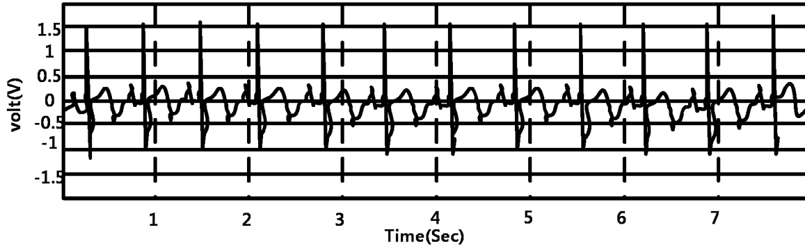
(a) 기준신호(Biopac) 심전계로 측정된 ECG
