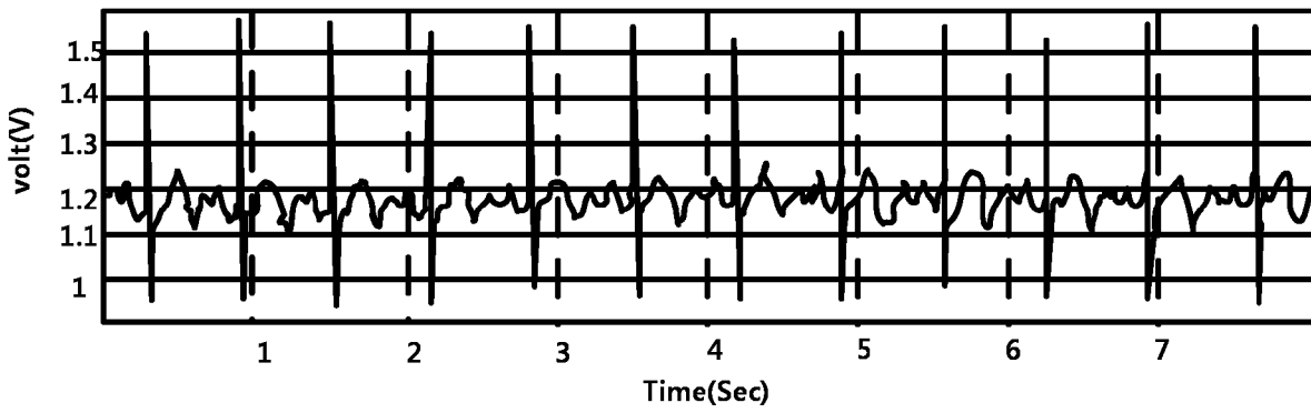
(b) savitzky-golay filter를 적용한 체중계형 심전계 ECG
