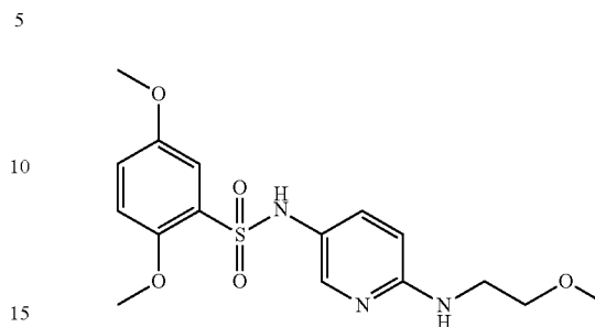
Example VIII-12: 2,5-Dimethoxy-N-(6-((2-methoxyethyl)amino)pyridin-3-yl)benzenesulfonamide
