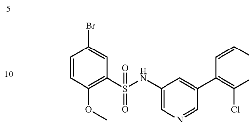
Example III-41: 5-Bromo-N-[5-(2-chloro-phenyl)-pyridin-3-yl]-2-methoxy-benzenesulfonamide
