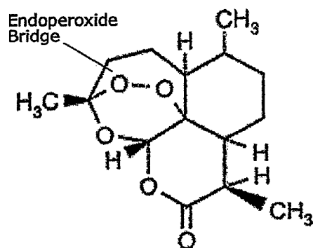
Artemisinin
