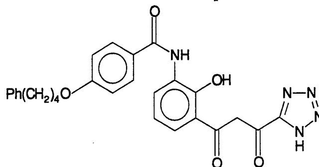
(IIA)
