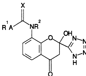
(IIB)
