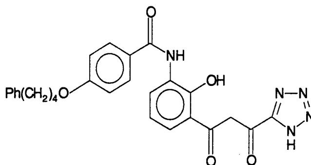
(IIA)
