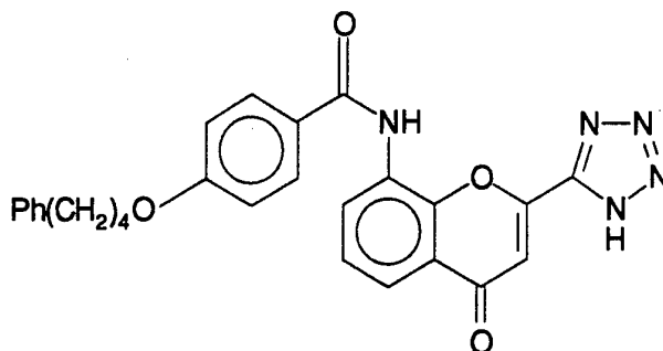
(IA)
