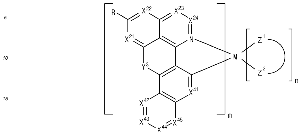
[Formula 1-5]
