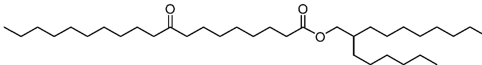
2-Hexyldecyl 9-oxononadecanoate
