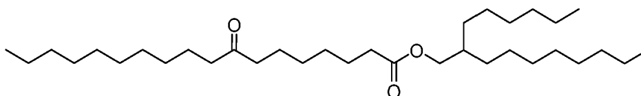
2-Hexyldecyl 8-oxooctadecanoate
