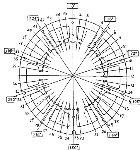
a 非対称型固定子構造
