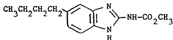
Parbendazole
