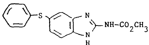
Fenbendazole
