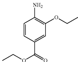
Ethyl 4-amino-3-ethoxybenzoate
