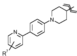
(1B-2)
