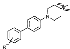
(1B-1)
