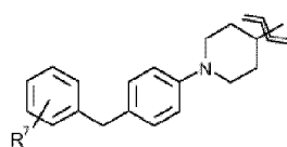
(1B-5)
