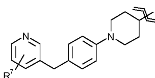
(1B-6)
