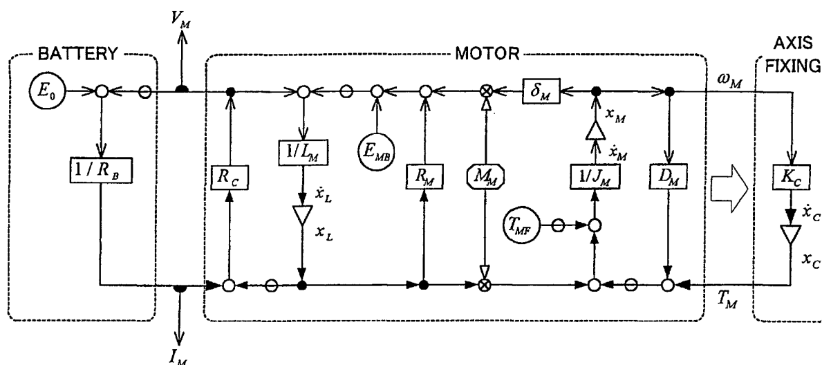
FIG.22
