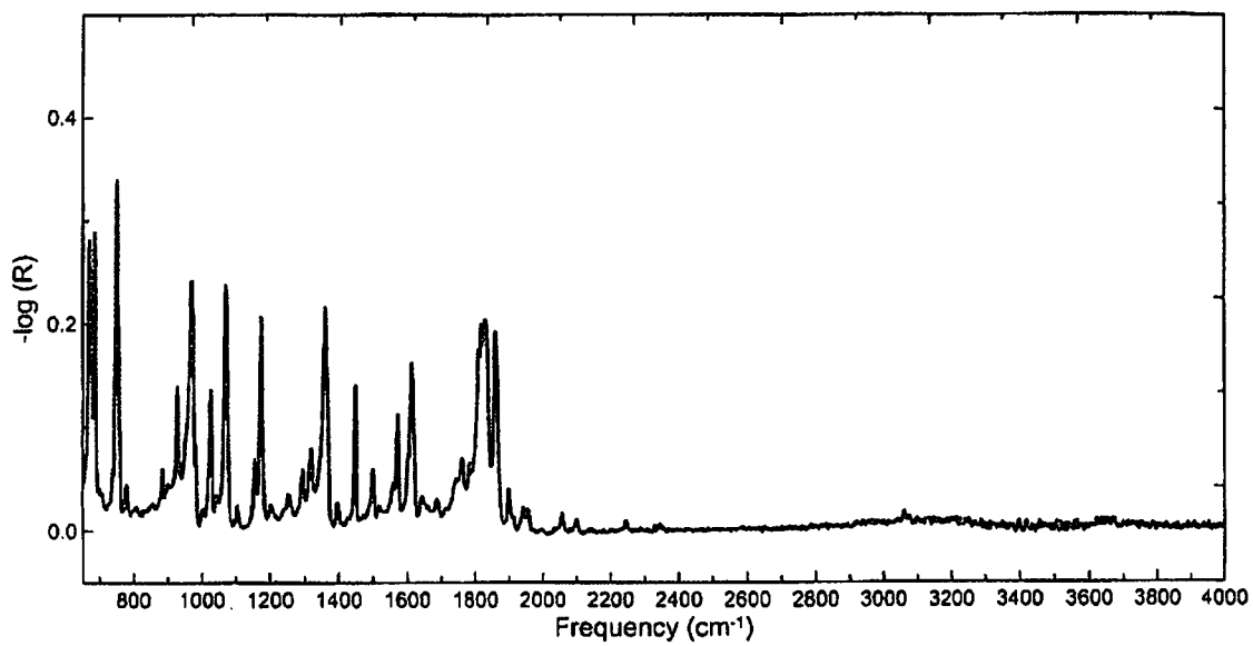
FIG. 9 FTIR spectrum of PDO.
