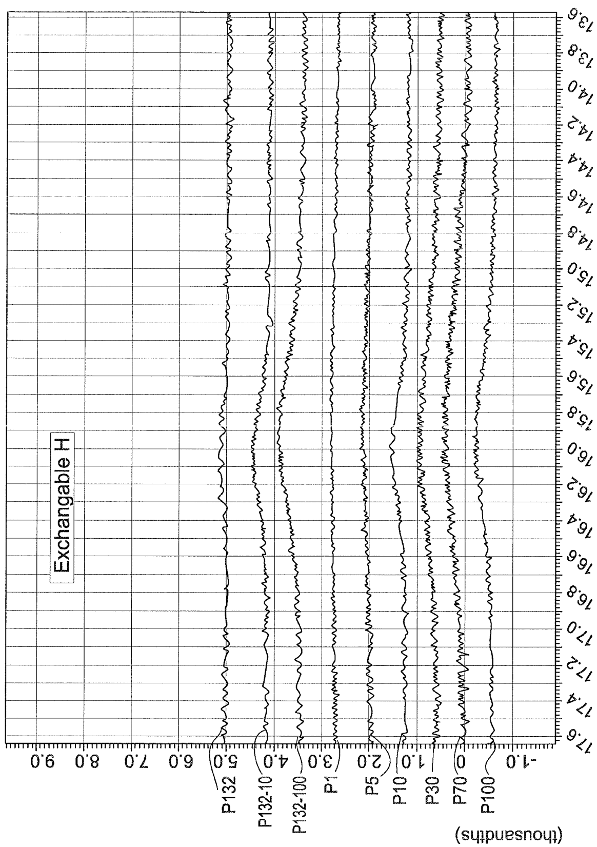
FIG. 38J X : parts per Million : 1H
