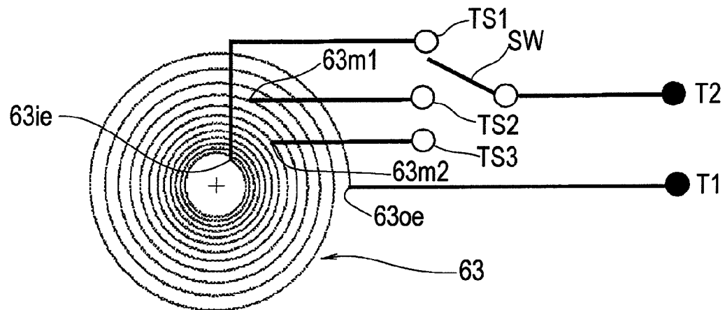
FIG. 22A
