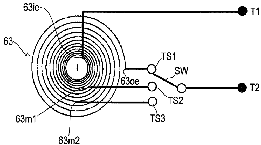
FIG. 22B
