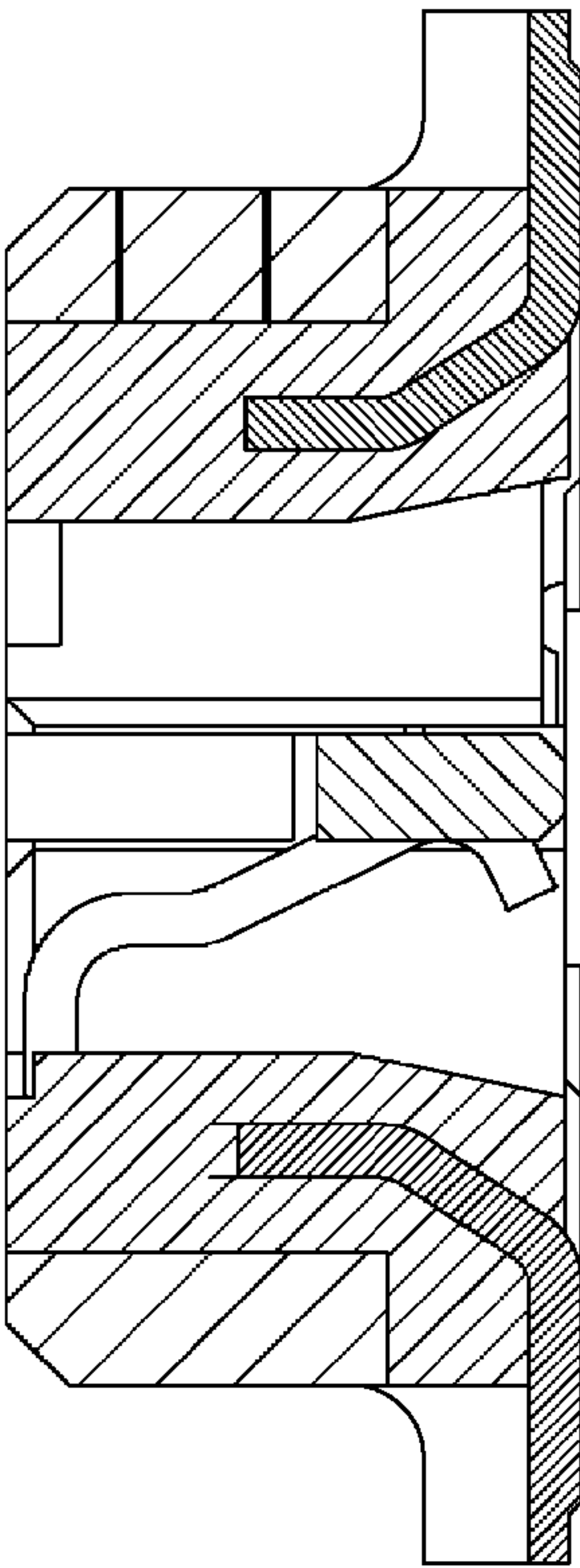
【 A－A剖面圖】
