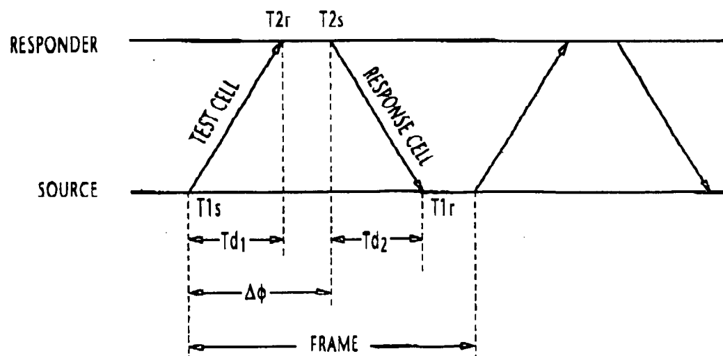
FIG. 8C HANDSHAKING MODE
