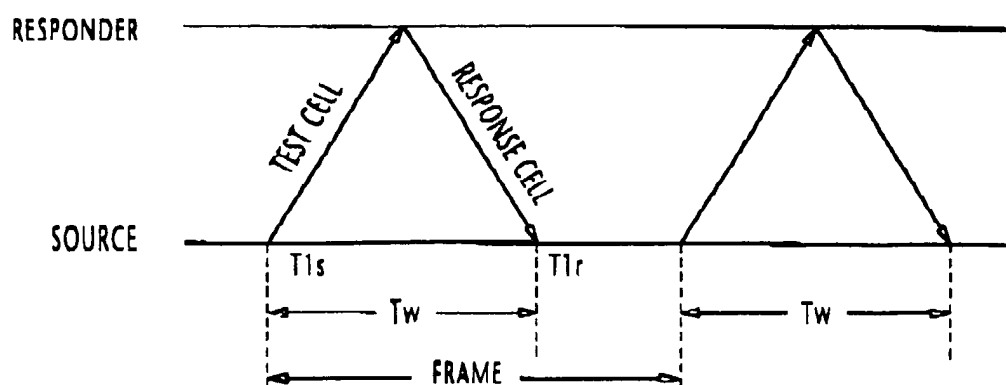
FIG. 8A LOOPBACK MODE
