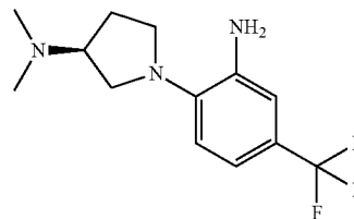
(S)-1-(2-amino-4-(trifluoromethyl)phenyl)-N,N-dimethylpyrrolidin-3-amine
