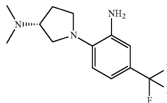
(R)-1-(2-amino-4-(trifluoromethyl)phenyl)-N,N-dimethylpyrrolidin-3-amine
