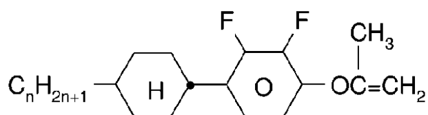
CY-n-OC(CH 3 )=CH 2
