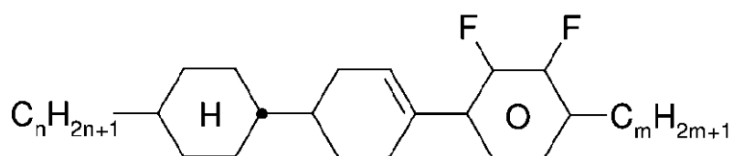
CLY-n-m
