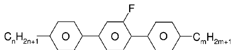
PGP-n-m
