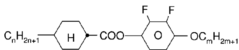
D-nOmFF
