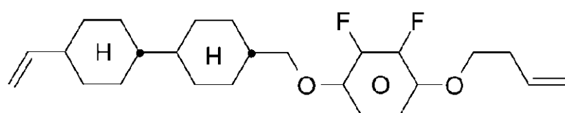
CCOY-V-O2V
