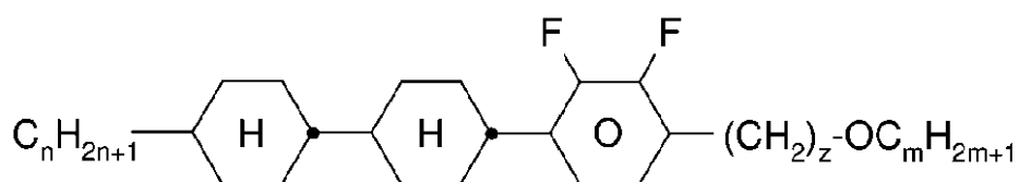
CCY-n-zOm
