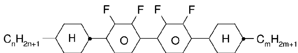
CYYC-n-m
