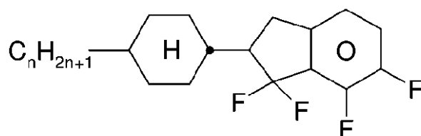
CK-n-F
