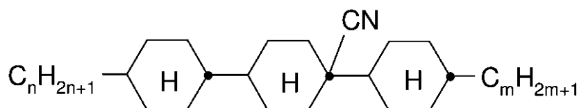
BCN-nm
