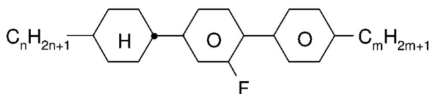
BCH-nmF
