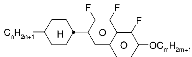
CNaph-n-Om
