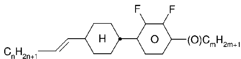
CY-nV-(O)m
