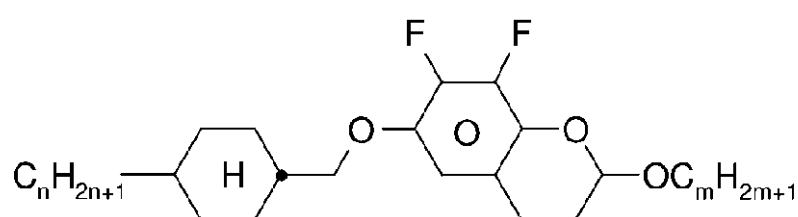
COChrom-n-Om
