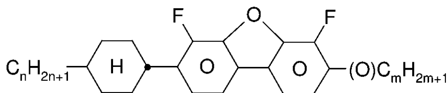
C-DFDBF-n-(O)m
