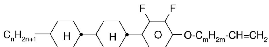
CCY-n-OmV
