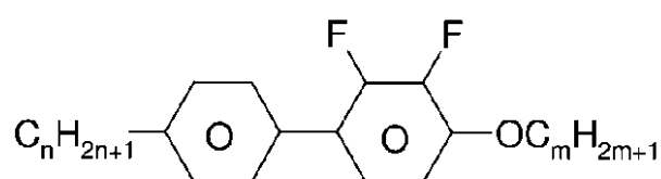
PY-n-Om
