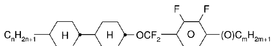
CCQIY-n-(O)m
