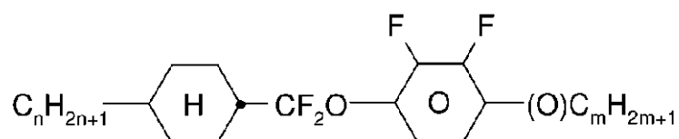
CQY-n-(O)m
