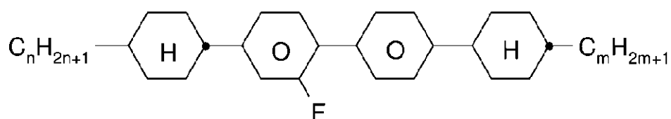
CBC-nmF
