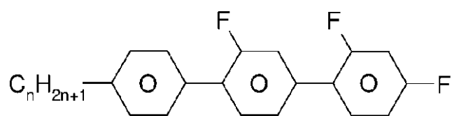
PGIGI-n-F
