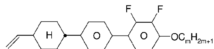
CPY-V-Om
