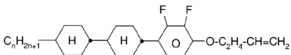
CCY-n-O2V
