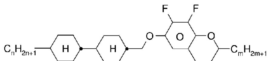
CCOChrom-n-m
