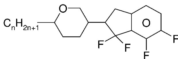
AIK-n-F
