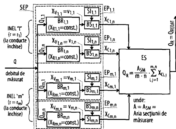
Fig. 3 Structura debitmetrelor multiinsertie - Schema structurală S2b
