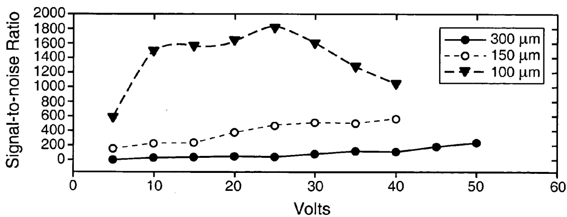
FIG. 9C
