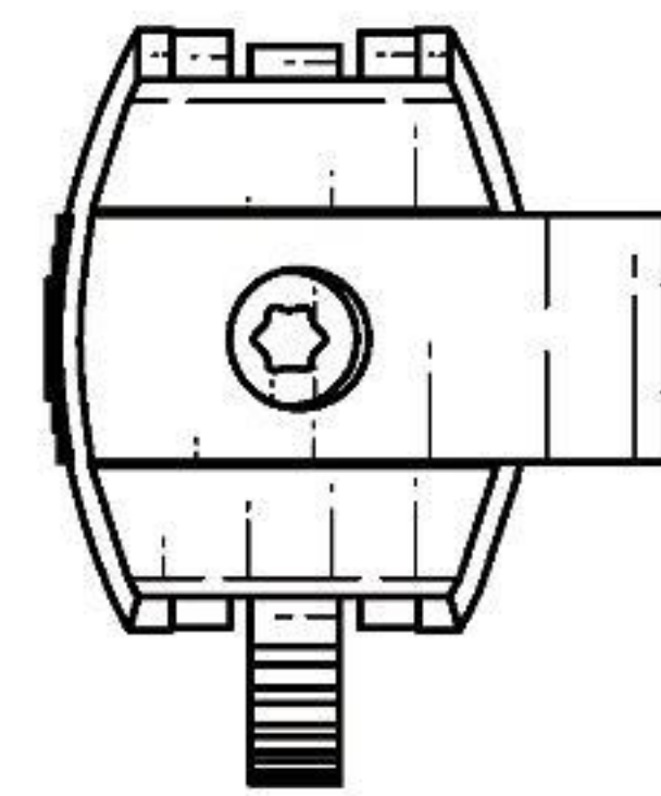
【右側視圖】
