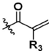
(meth)acryl
