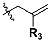
(meth)allyl
