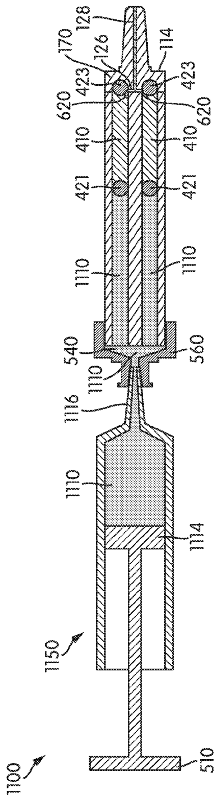
FIG. 11C
