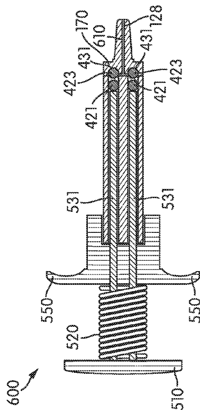
FIG. 6D
