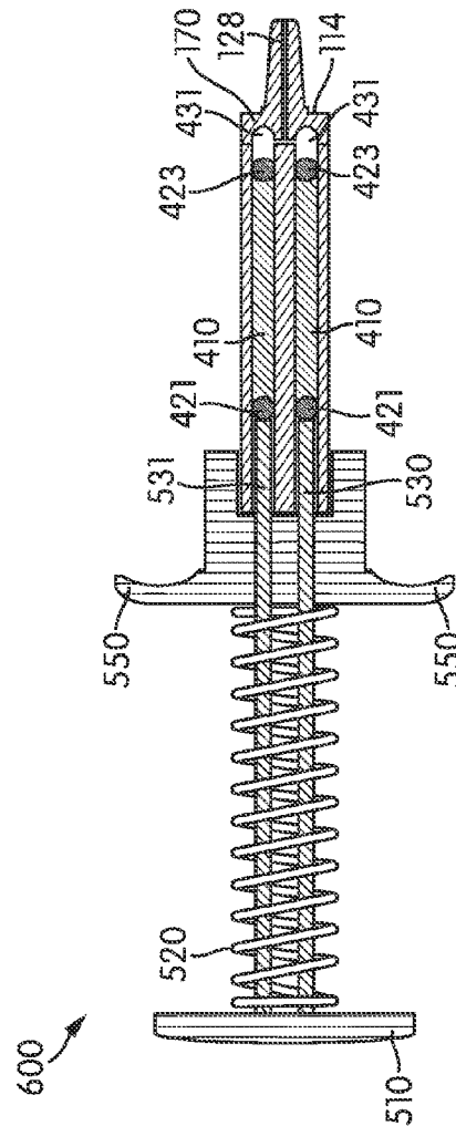
FIG. 6B
