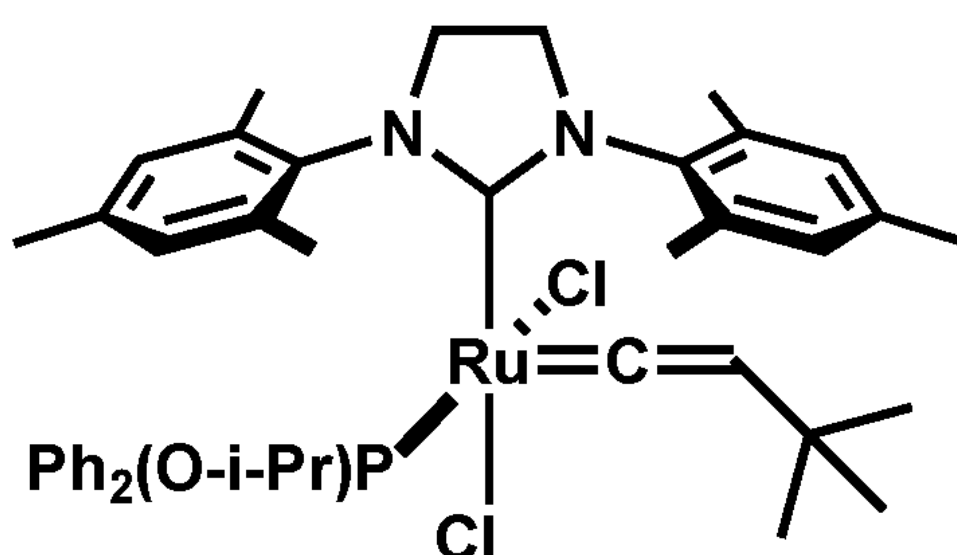
cis-C805v
