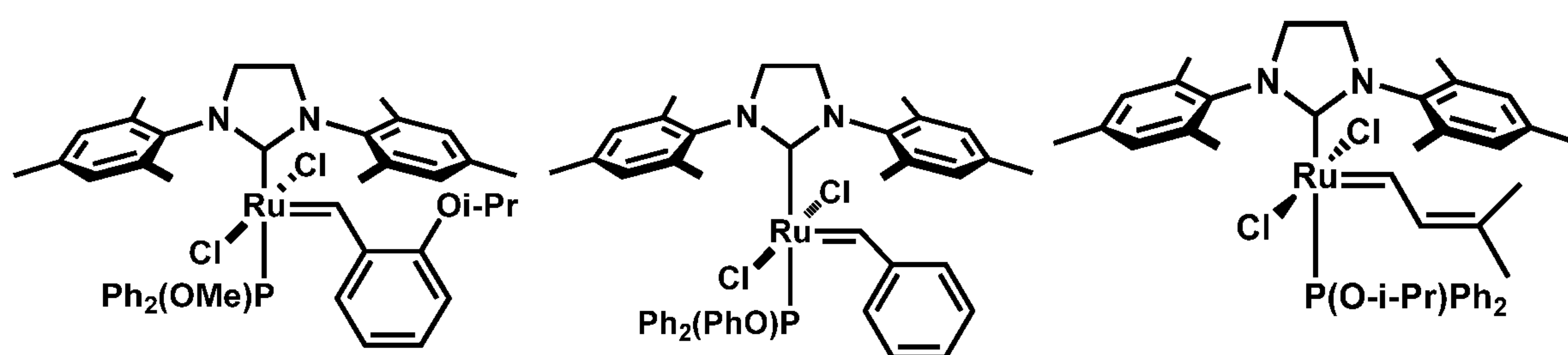
trans -C843
