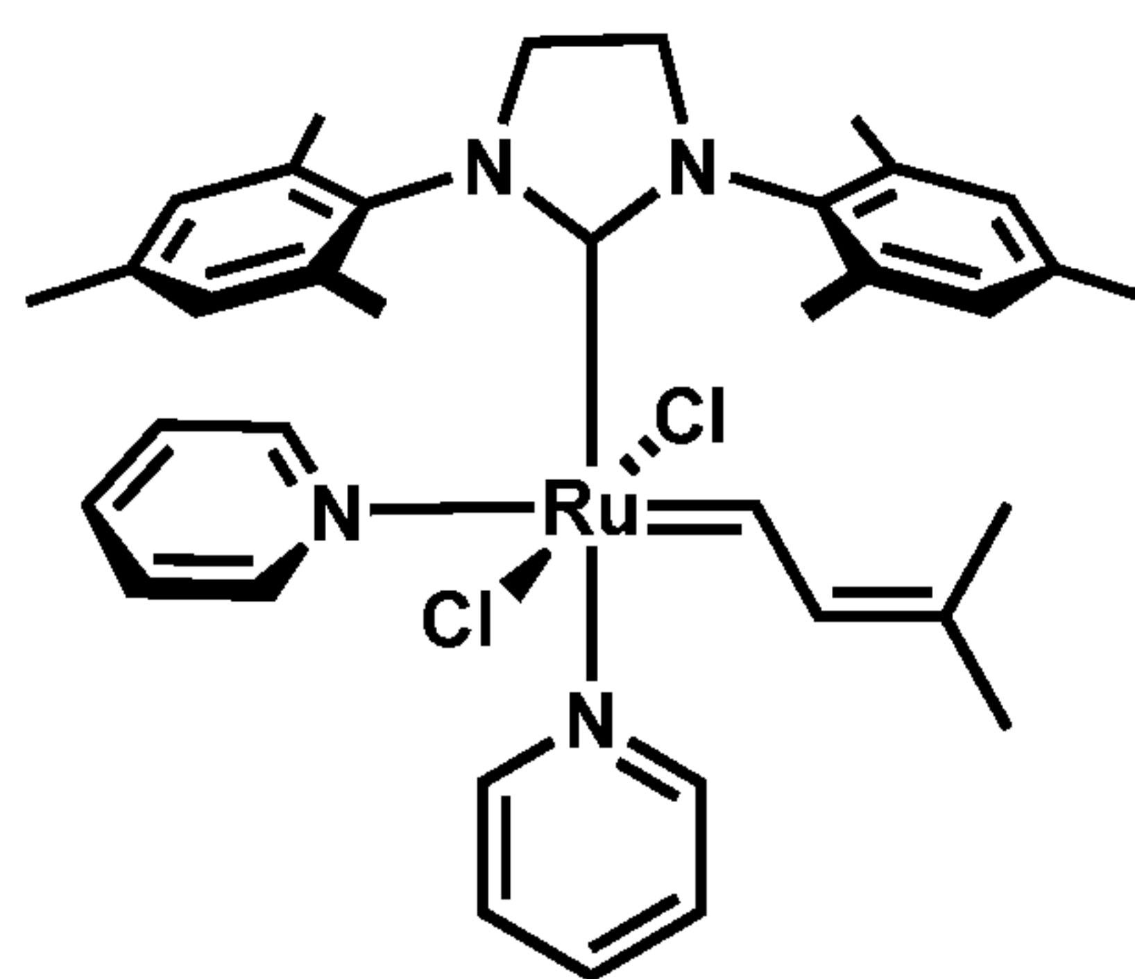
trans-C705
