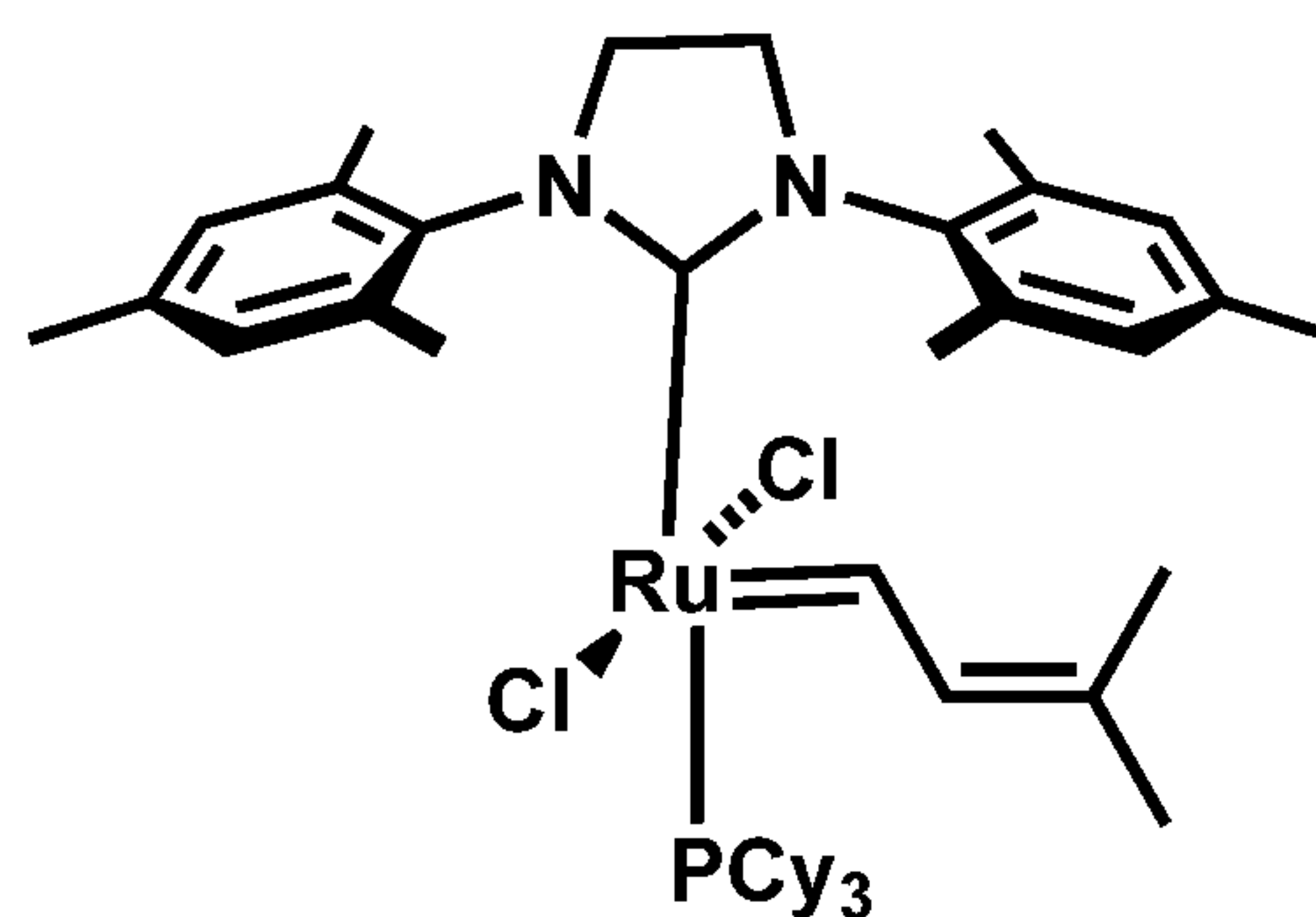
trans-C827
