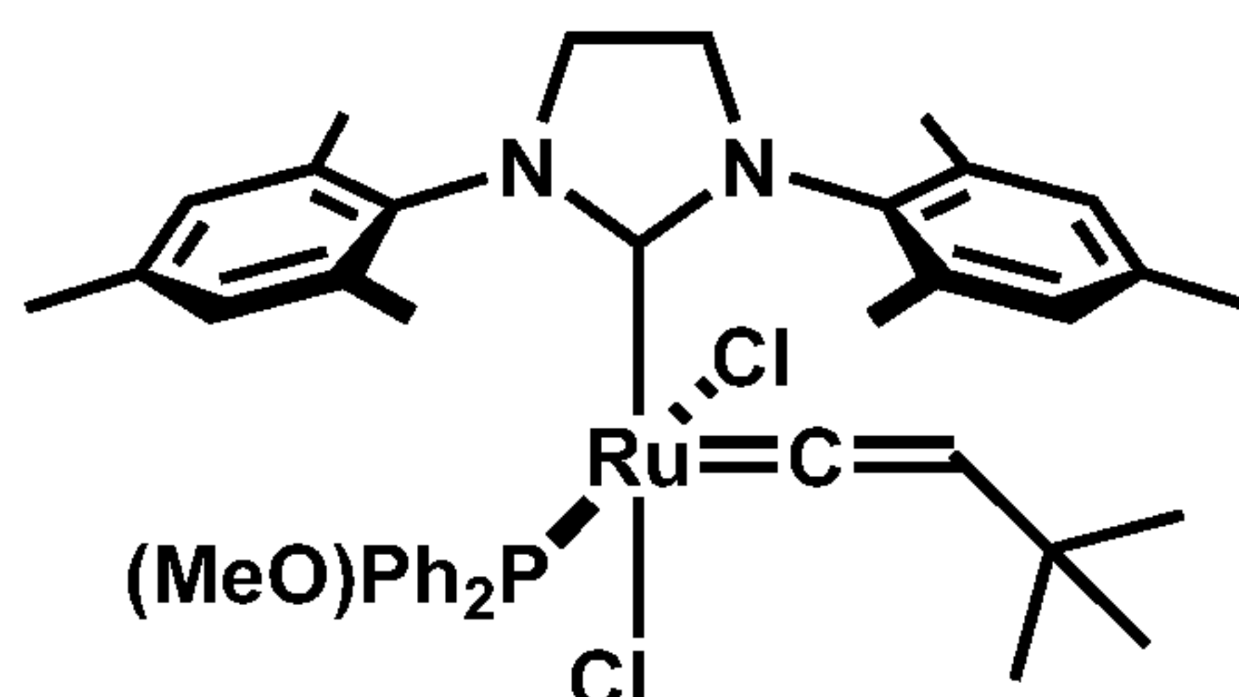
cis -C777v
