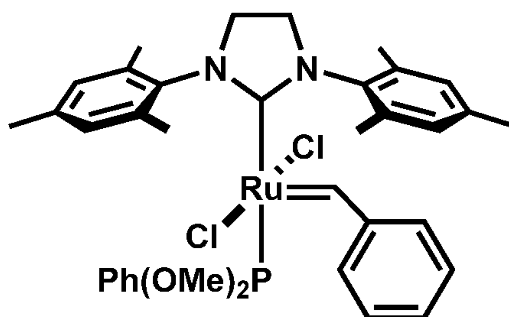
trans-C739
