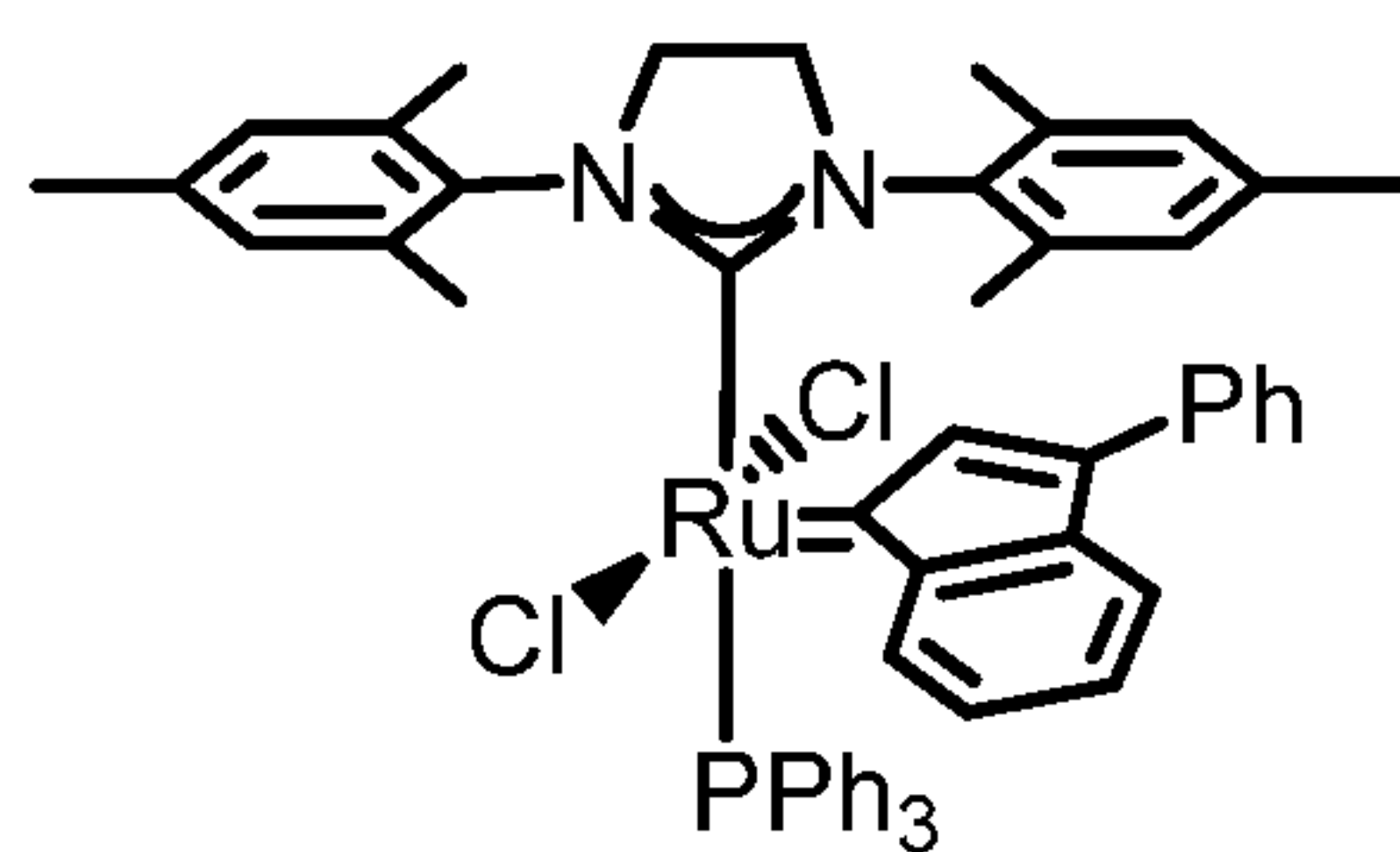
(III)
