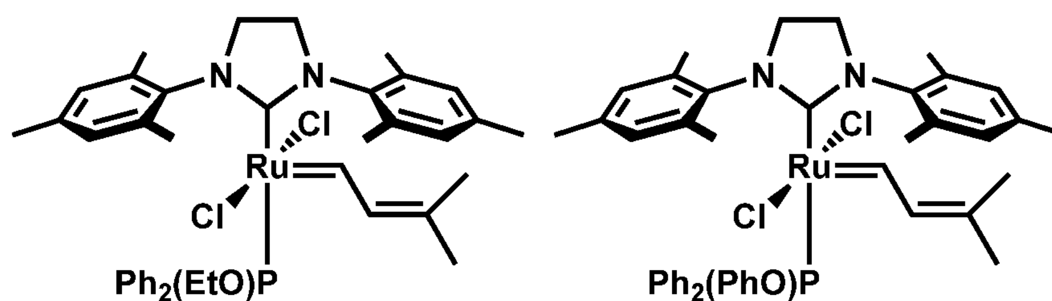
trans -C777
