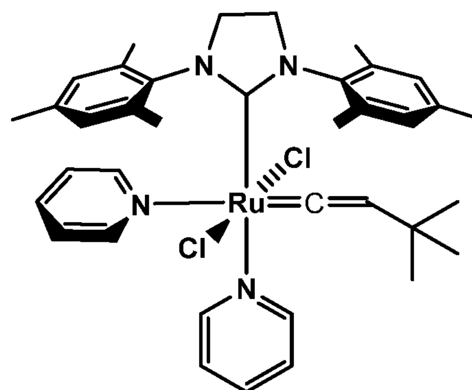
trans-C719v
