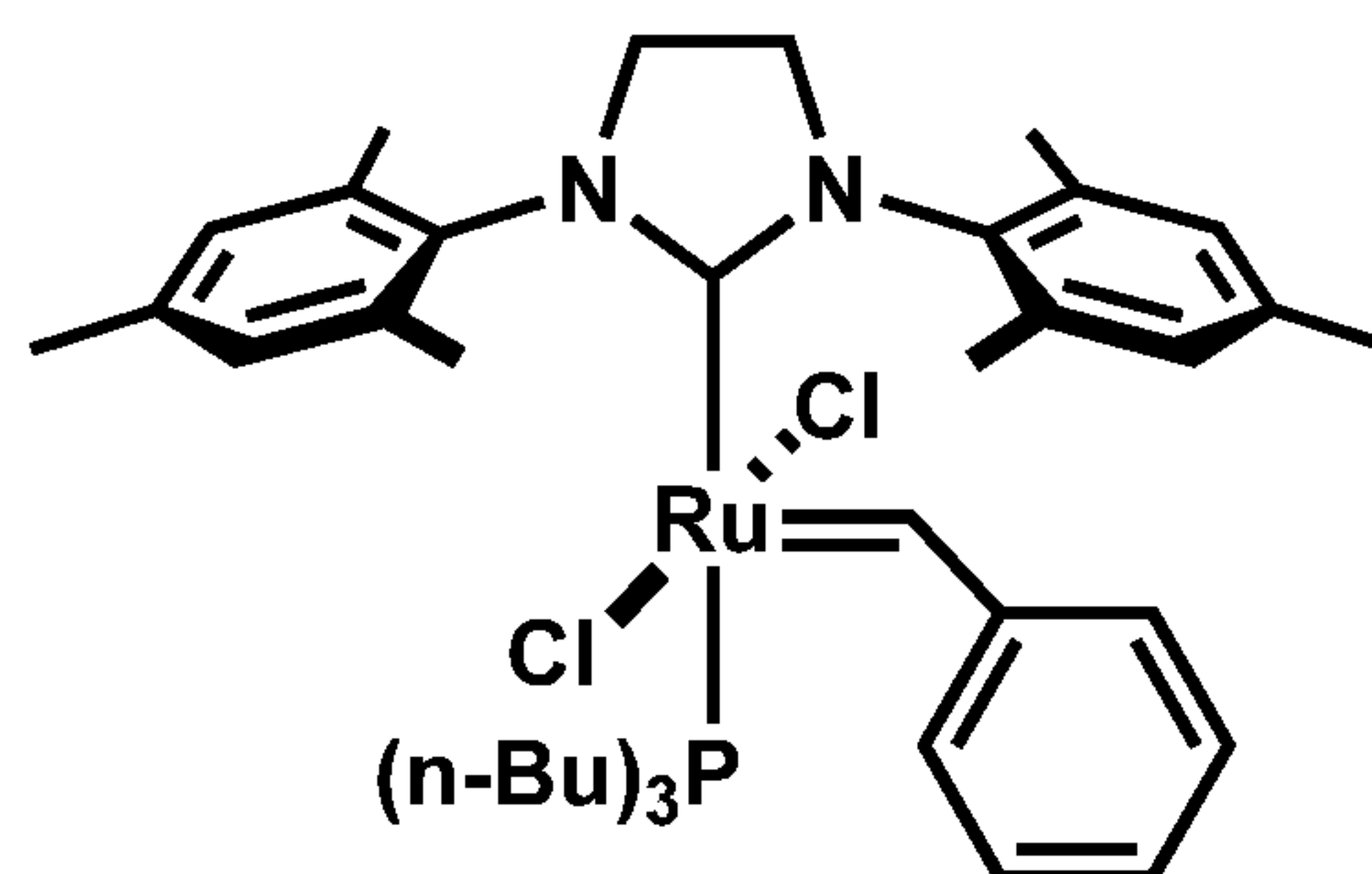
trans -C771
