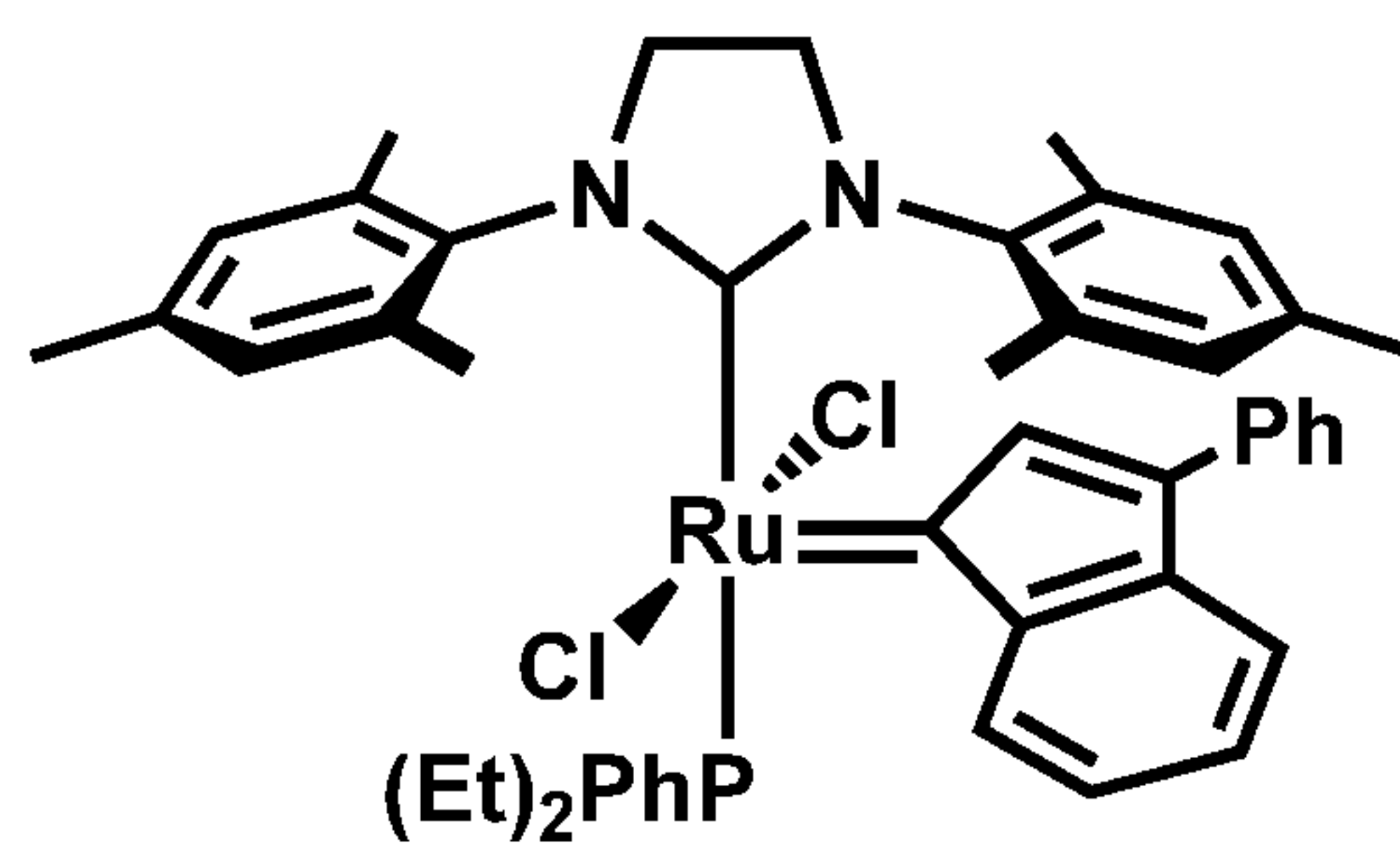
trans -C771
