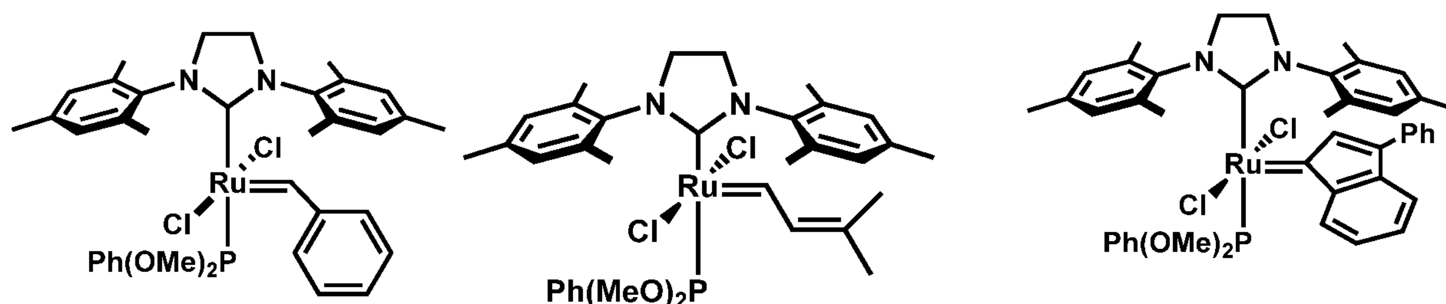
trans -C739
