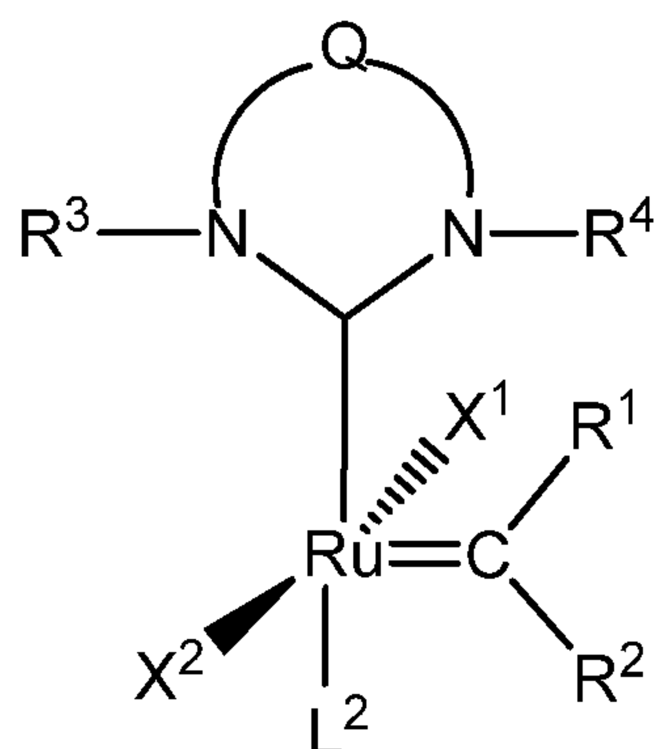
Formula (Va)
