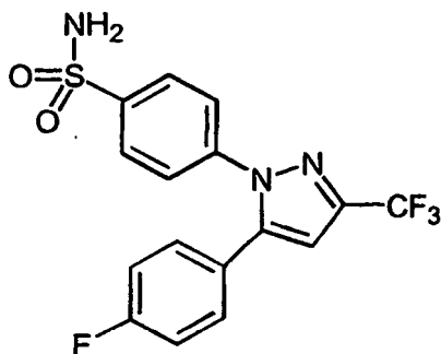
4-[5-(4-fluorophenyl)-3-(trifluoromethyl)-1H-pyrazol-1-yl]benzenesulfonamide; C18)
