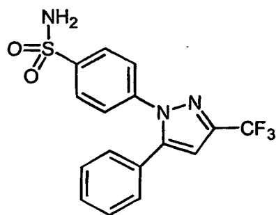
4-[5-phenyl]-3-(trifluoromethyl)-1H-pyrazol-1-yl]benzenesulfonamide; C16)
