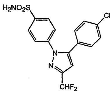
4-[5-(4-chlorophenyl)-3-(difluoromethyl)-1H-pyrazol-1-yl]benzenesulfonamide; C20)
