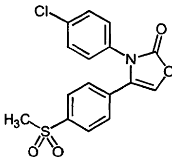
3-(4-chlorophenyl)-4-[4-(methylsulfonyl)phenyl]-2-(3H)-oxazolone; C10)
