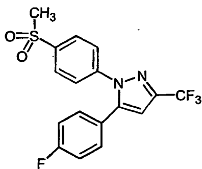
5-(4-fluorophenyl)-1-[4-(methylsulfonyl)phenyl]-3-(trifluoromethyl)-1H-pyrazole; C15)
