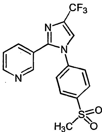
3-[1-[4-(methylsulfonyl)phenyl]-4-(trifluoromethyl)-1H-imidazol-2-yl]pyridine; C21)
