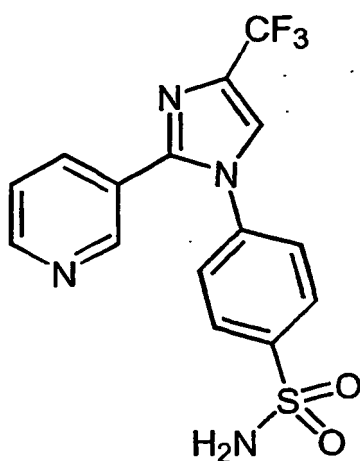
4-[2-(3-pyridinyl)-4-(trifluoromethyl)-1H-imidazol-1-yl]benzenesulfonamide; C22)
