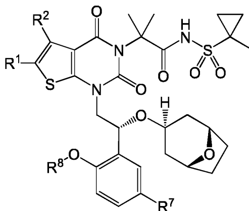
(IVa).
