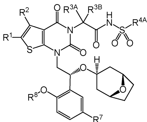
Formel (IIIa).
