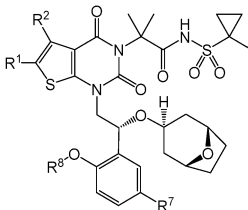
Formula (IVa).
