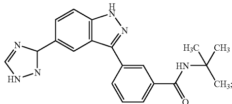
N-tert-Butyl-3-[5-(1H-[1,2,4]triazol-3-yl)-1H-indazol-3-yl]-benzamide
