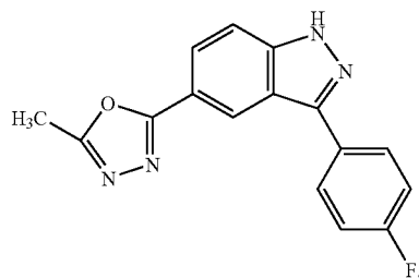
3-(4-Fluoro-phenyl)-5-(5-methyl-[1,3,4]oxadiazol-2-yl)-1H-indazole
