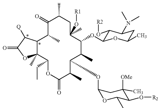
Formula I-a
