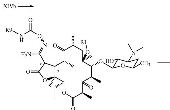
XVI
