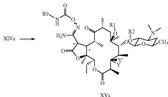
XVa
