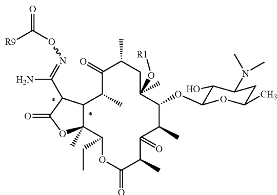
XIIb
