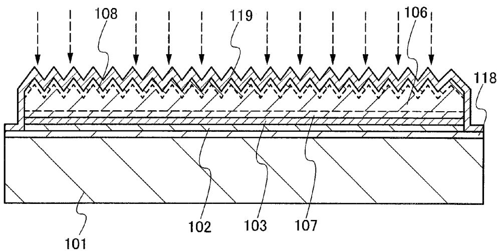
FIG. 18C
