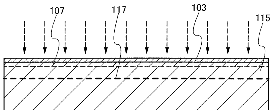
FIG. 12C
