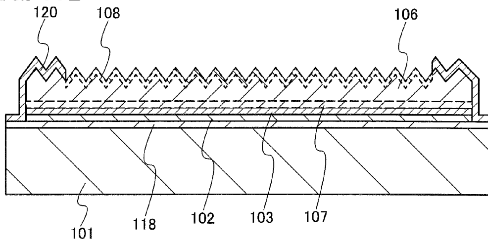
FIG. 19C
