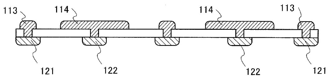
FIG. 20B
