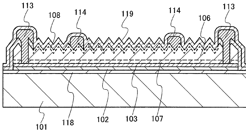
FIG. 19C
