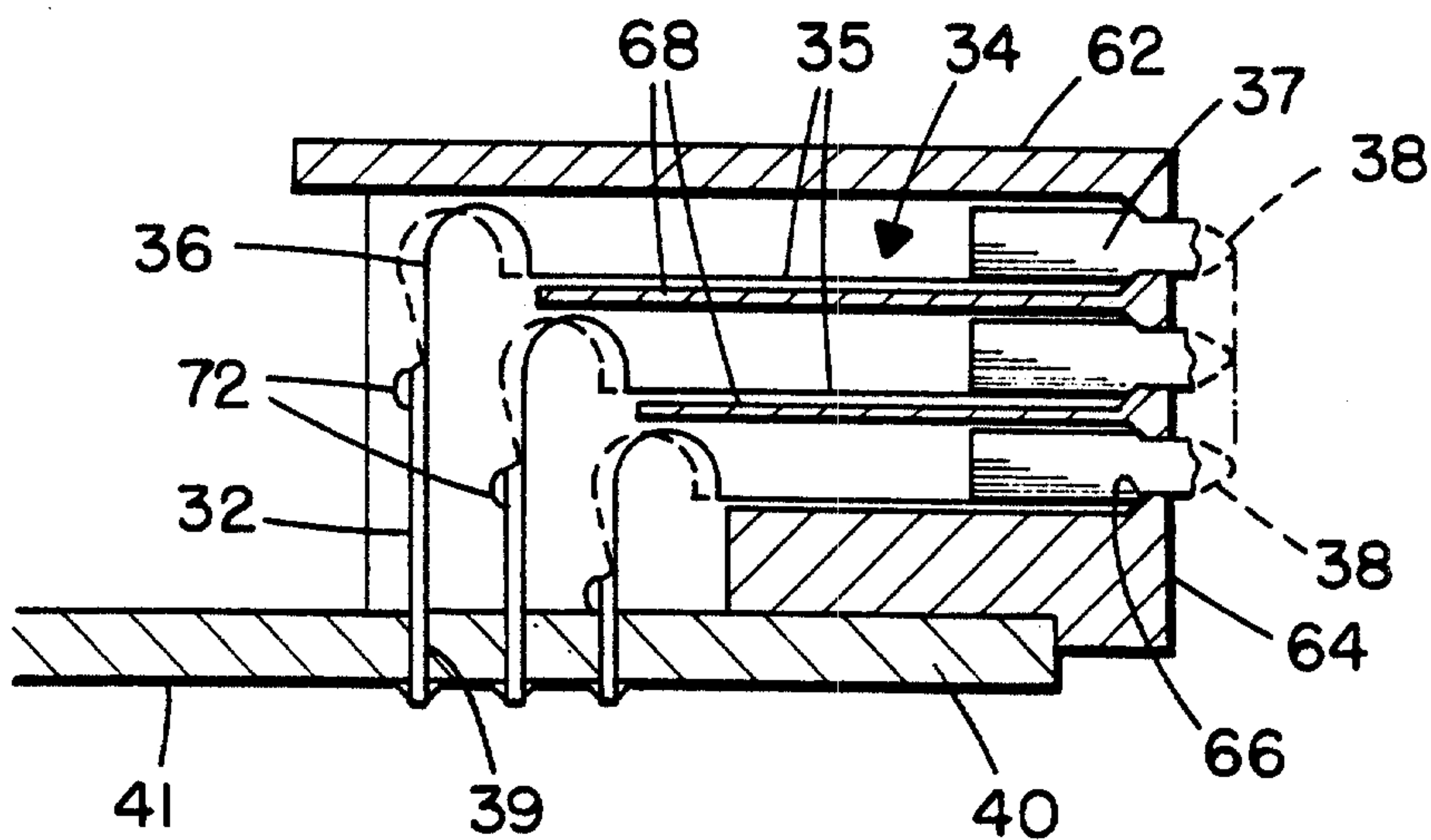
FIG. 3A.
