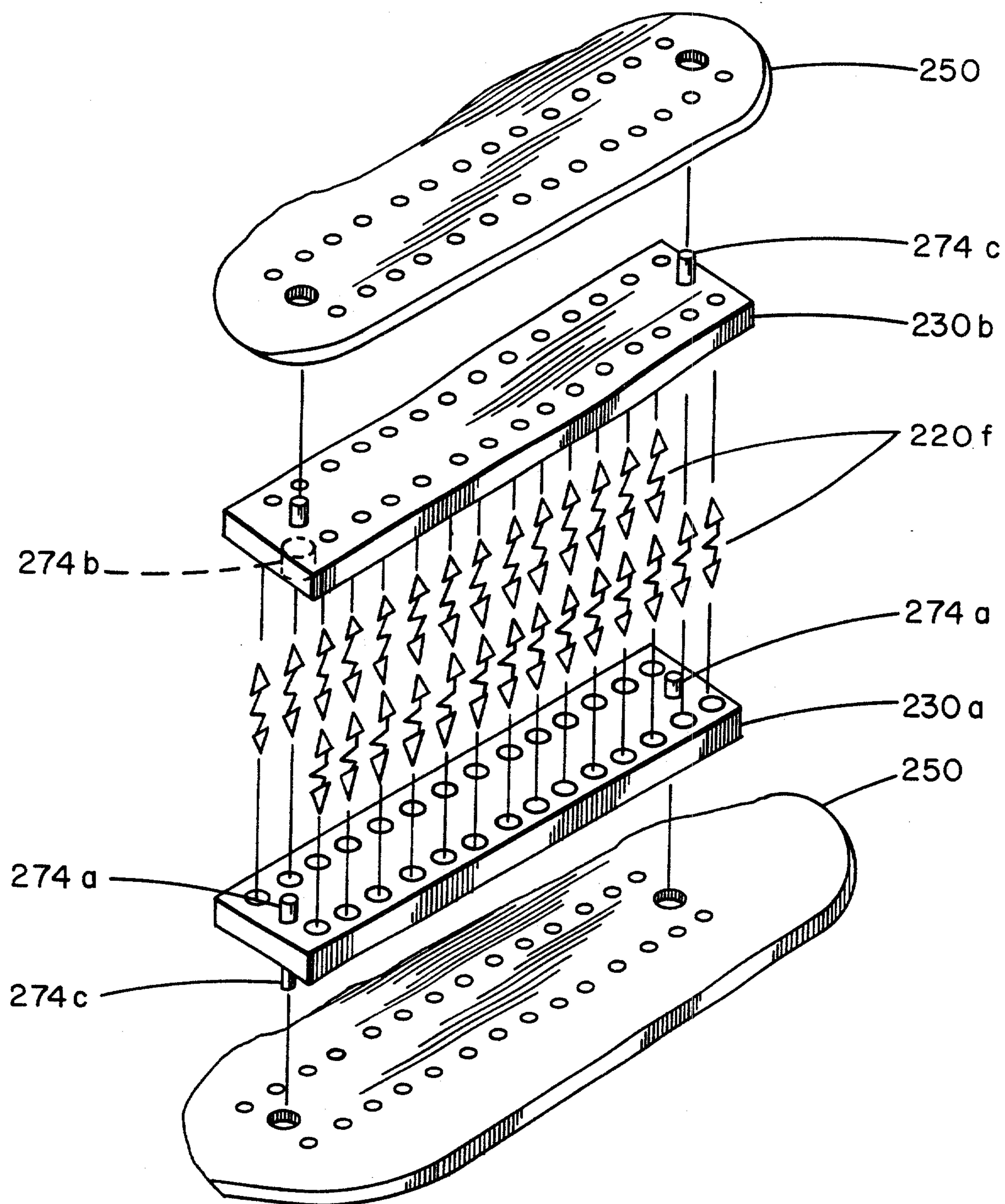
FIG. 5g
