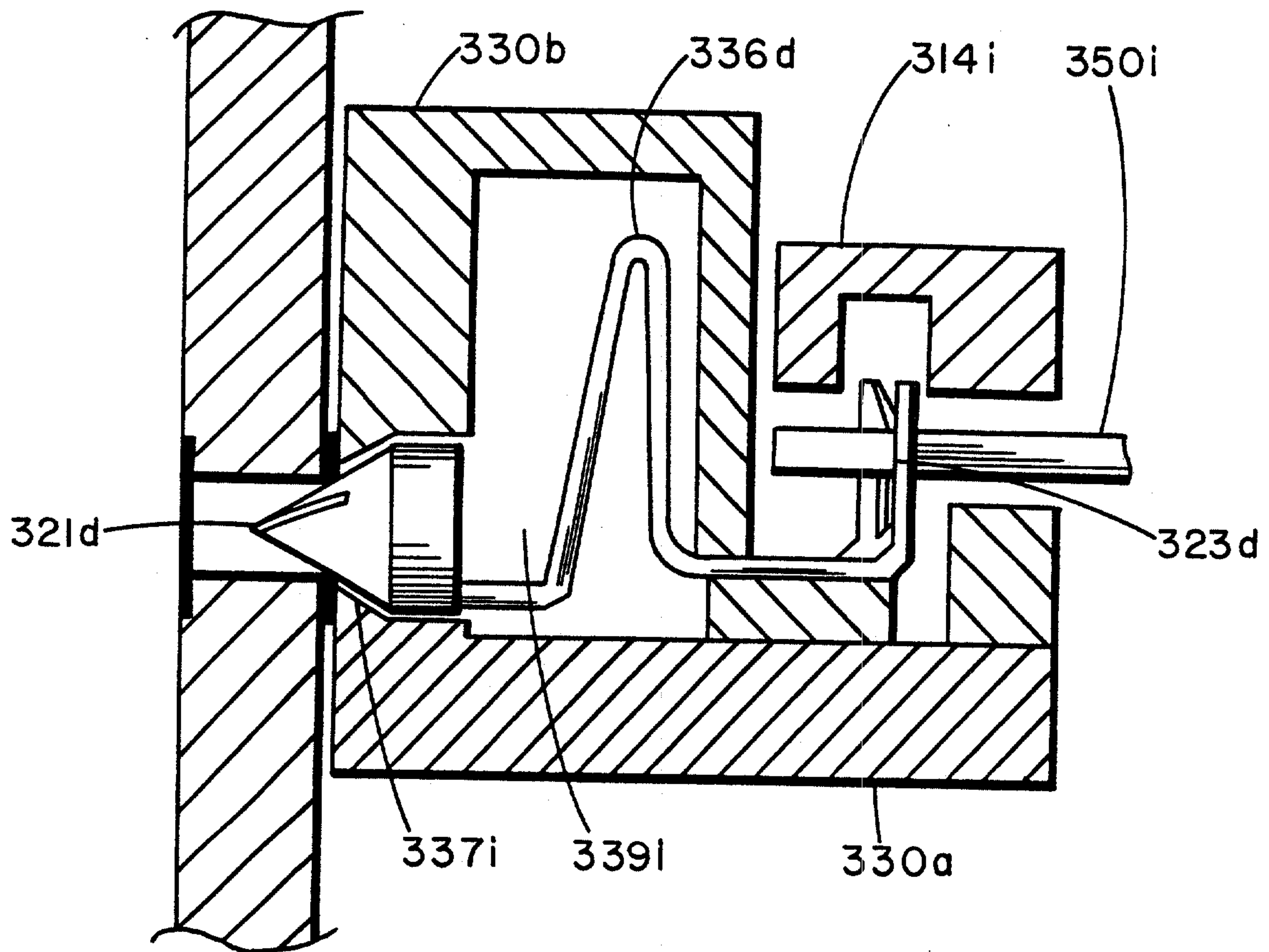
FIG. 6i
