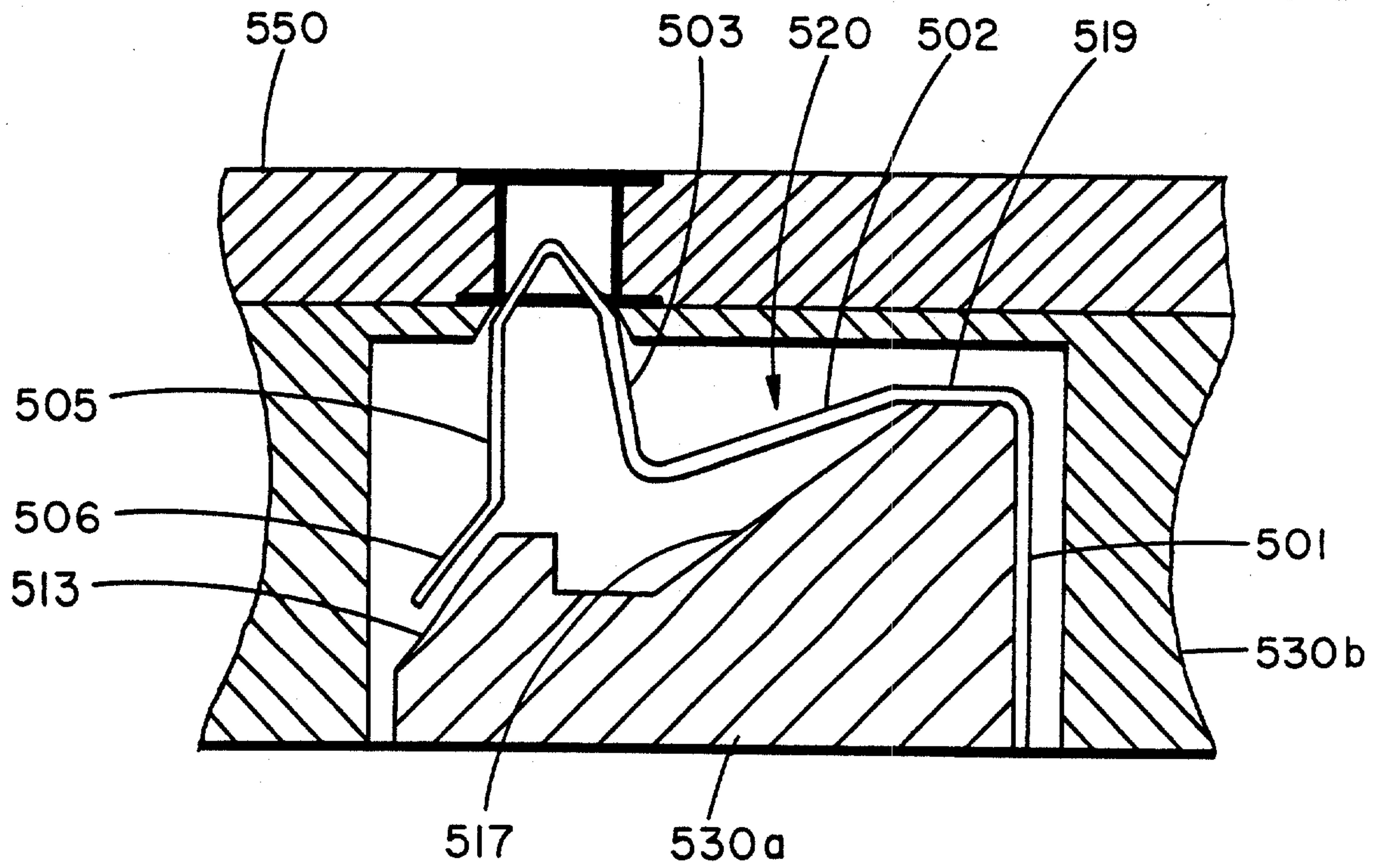
FIG. 8
