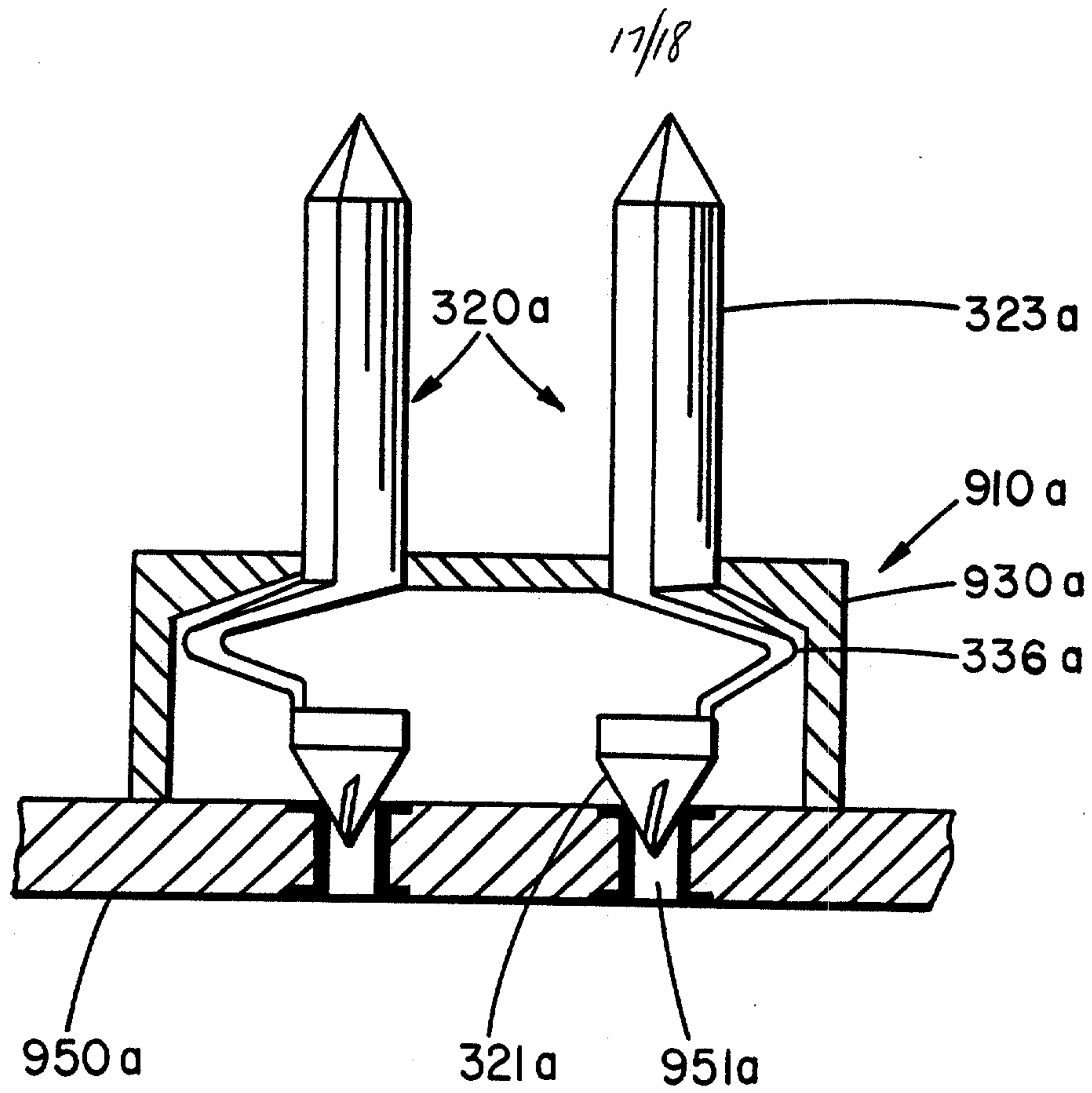
FIG. 12 a
