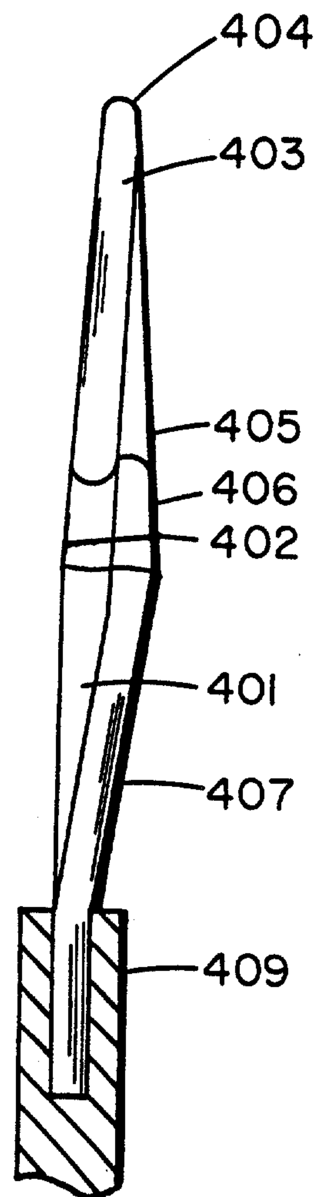
FIG. 7b
