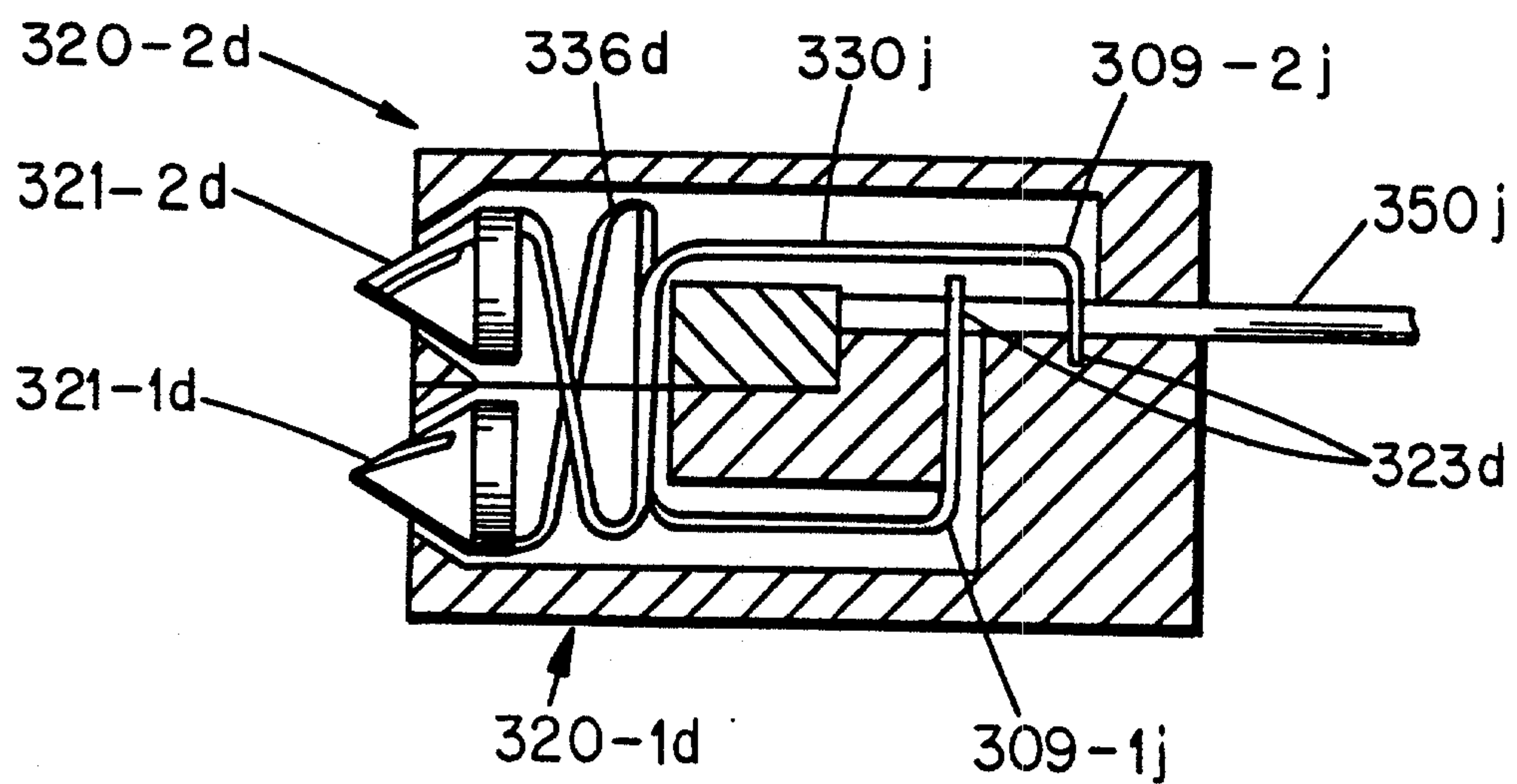
FIG. 6j
