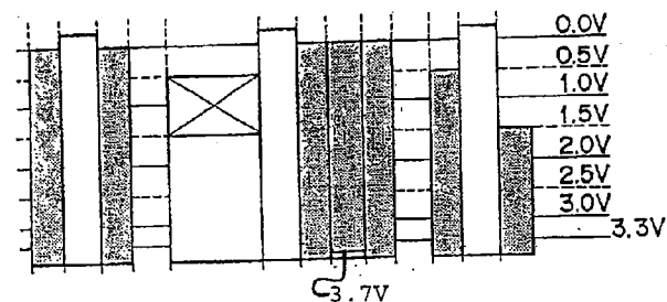
FIG. 15D t_3 < t < t_4
