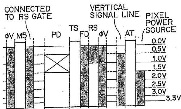
FIG. 15B t_1 < t < t_2
