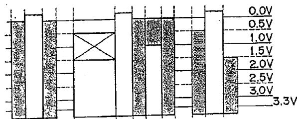
FIG. 15B t_1 < t < t_2
