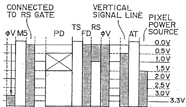
FIG. 16A t_4 < t < t_5
