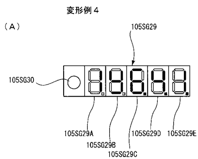
(B) 7セグ+ドット
