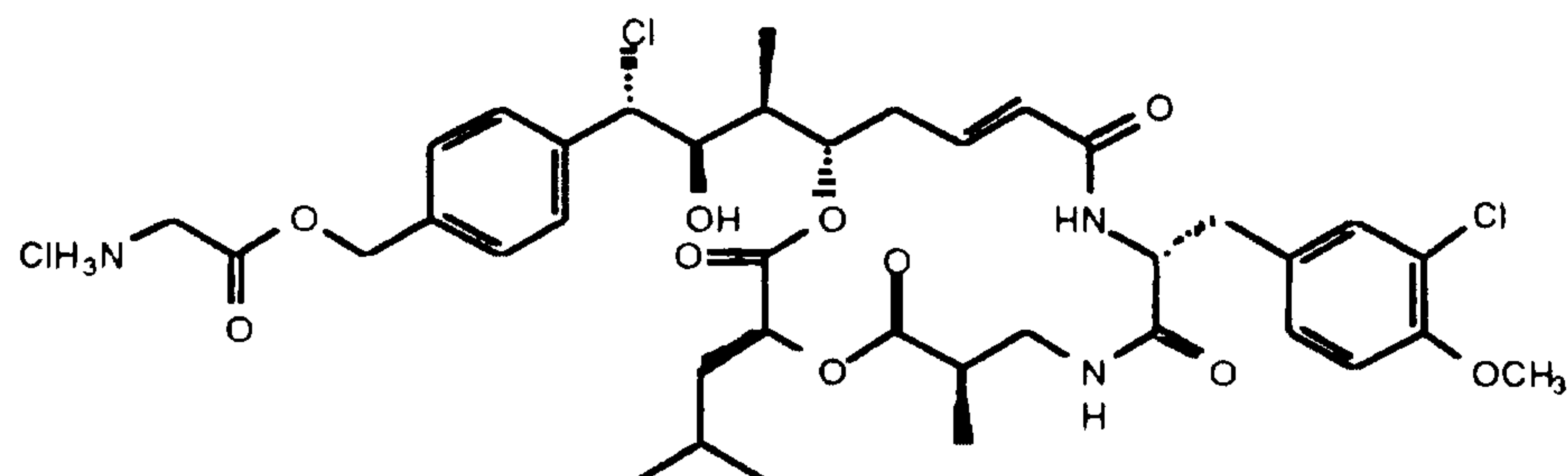
Cryptophycin-273
