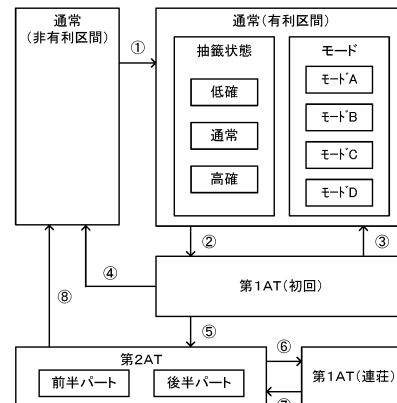
(C) 遷移条件
