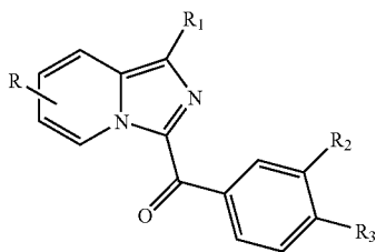
(Iy)
