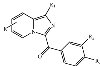
(Iw)
