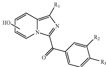
(Iz)
