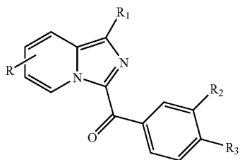
(Iu)
