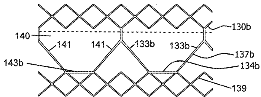
FIG. 7B
