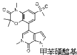
化合物8，
