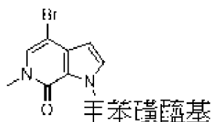
化合物9
