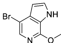
化合物12
