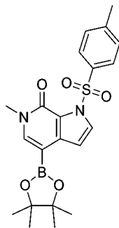
化合物15
