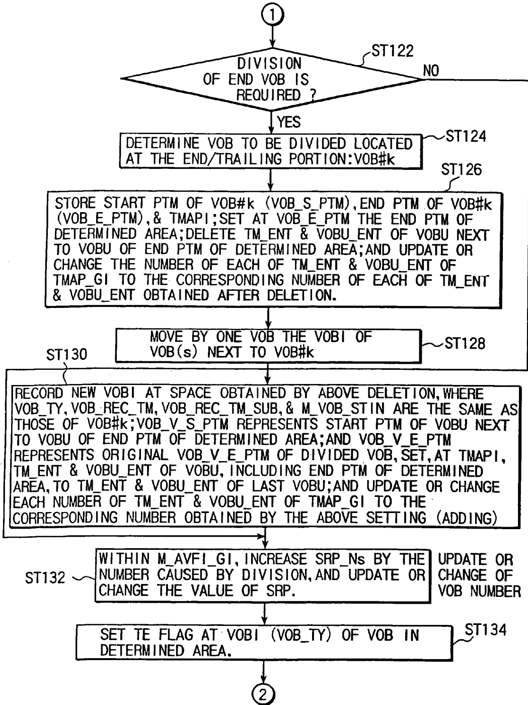
FIG. 46
