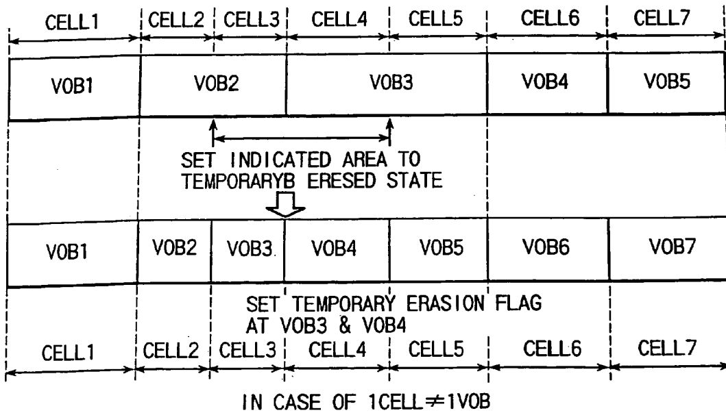
FIG. 50
