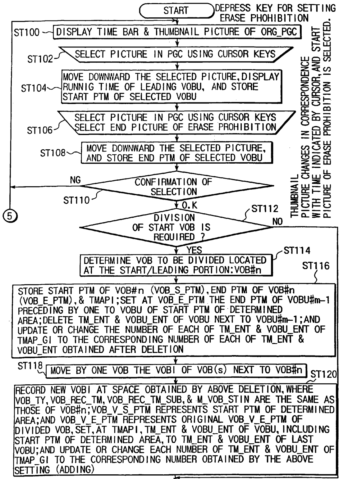
FIG. 45
