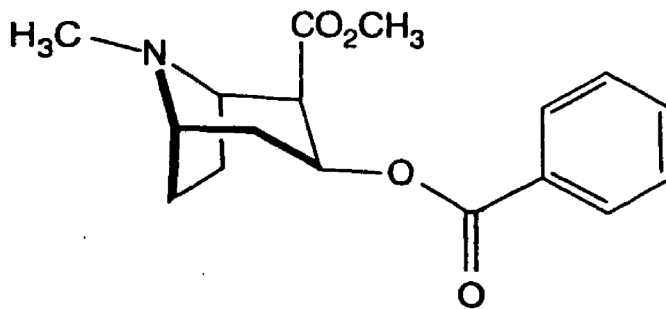
(-)-COCAINE FIG. 1A
