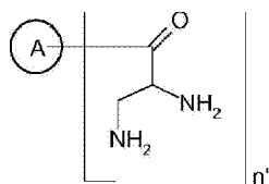
(II-b)
