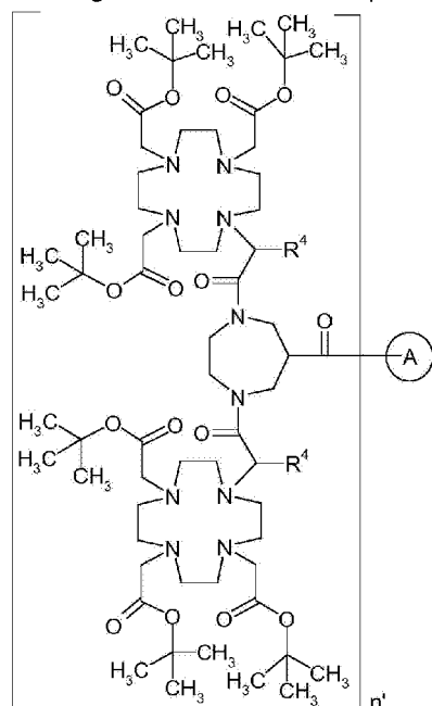
(V)
