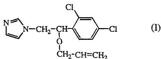
imazalil
