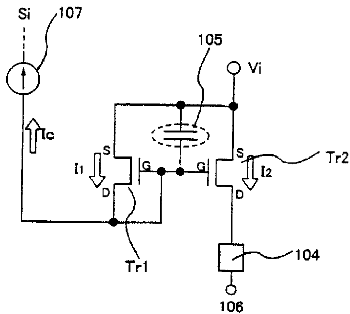
FIG. 4B DISPLAY PERIOD T_d
