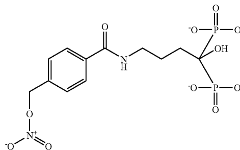
NOX-alendronate
