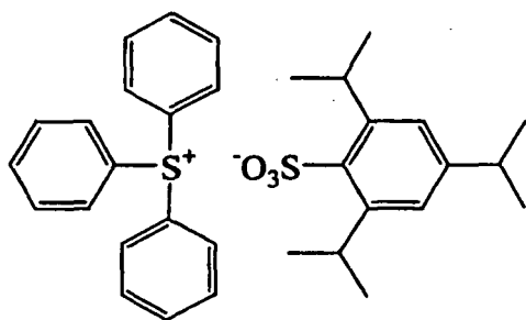
PAG-1
