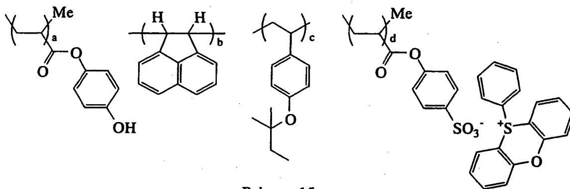
Polymer 15 (C-NMR ratio, a : b : c : d = 50 : 10 : 37 : 3)
