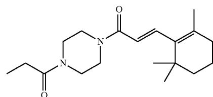
(E)-1-(4-Propionylpiperazin-1-yl)-3-(2,6,6-trimethylcyclohex-1-enyl)prop-2-en-1-one
