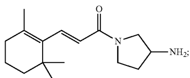
(E)-1-(3-Aminopyrrolin-1-yl)-3-(2,6,6-trimethylcyclohex-1-enyl)prop-2-en-1-one
