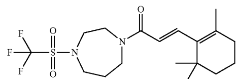
(E)-1-(4-(Trifluoromethylsulfonyl)-1,4-diazepan-1-yl)-3-(2,6,6-trimethylcyclohex-1-en-1-yl)prop-2-en-1-one
