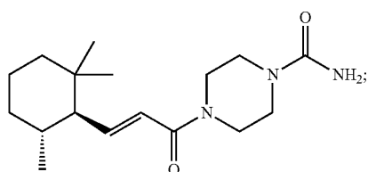
(-)-4-((E)-3-((1R,6R)-2,2,6-trimethylcyclohexyl)acryloyl)piperazine-1-carboxamide
