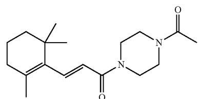
(E)-1-(4-Acetylpiperazin-1-yl)-3-(2,6,6-trimethylcyclohex-1-enyl)prop-2-en-1-one
