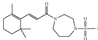
(E)-1-(4-(Methylsulfonyl)-1,4-diazepan-1-yl)-3-(2,6,6-trimethylcyclohex-1-en-1-yl)prop-2-en-1-one
