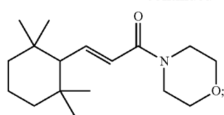
(E)-1-Morpholino-3-(2,2,6,6-tetramethylcyclohexyl)prop-2-en-1-one
