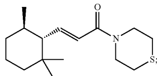
(E)-1-Thiomorpholino-3-((1R,6R)-2,2,6-trimethylcyclohexyl)prop-2-en-1-one
