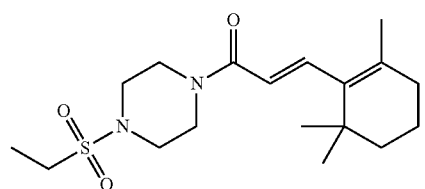
(E)-1-(4-(Ethylsulfonyl)piperazin-1-yl)-3-(2,6,6-trimethylcyclohex-1-en-1-yl)prop-2-en-1-one
