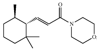
(E)-1-Morpholino-3-((1R,6R)-2,2,6-trimethylcyclohexyl)prop-2-en-1-one
