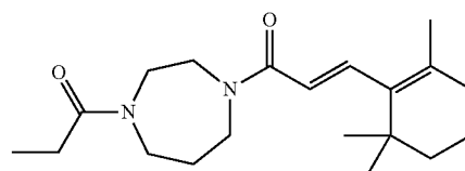
(E)-1-(4-Propionyl-1,4-diazepan-1-yl)-3-(2,6,6-trimethylcyclohex-1-en-1-yl)prop-2-en-1-one
