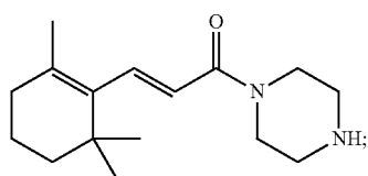
(E)-1-(Piperazin-1-yl)-3-(2,6,6-trimethylcyclohex-1-enyl)prop-2-en-1-one
