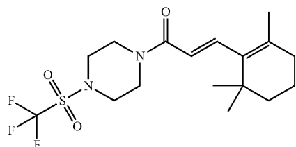
(E)-1-(4-(Trifluoromethylsulfonyl)piperazin-1-yl)-3-(2,6,6-trimethylcyclohex-1-en-1-yl)prop-2-en-1-one
