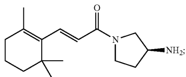
(W,E)-1-(3-Aminopyrrolidine-1-yl)-3-(2,6,6-trimethylcyclohex-1-en-1-yl)prop-2-en-1-one
