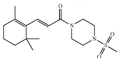
(E)-1-(4-(Methylsulfonyl)piperazin-1-yl)-3-(2,6,6-trimethylcyclohex-1-en-1-yl)prop-2-en-1-one
