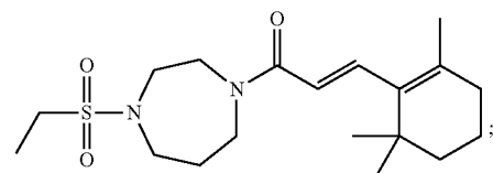
(E)-1-(4-(Ethylsulfonyl)-1,4-diazepan-1-yl)-3-(2,6,6-trimethylcyclohex-1-en-1-yl)prop-2-en-1-one
