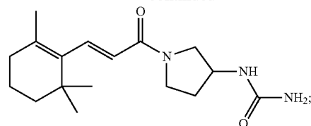
(E)-1-(3-(2,6,6-Trimethylcyclohex-1-enyl)acryloyl)-3-yl)urea
