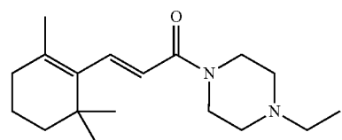
(E)-1-(4-Ethylpiperazin-1-yl)-3-(2,6,6-trimethylcyclohex-1-enyl)prop-2-en-1-one
