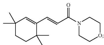
(E)-1-Morpholino-3-(3,3,6,6-tetramethylcyclohex-1-enyl)prop-2-en-1-one
