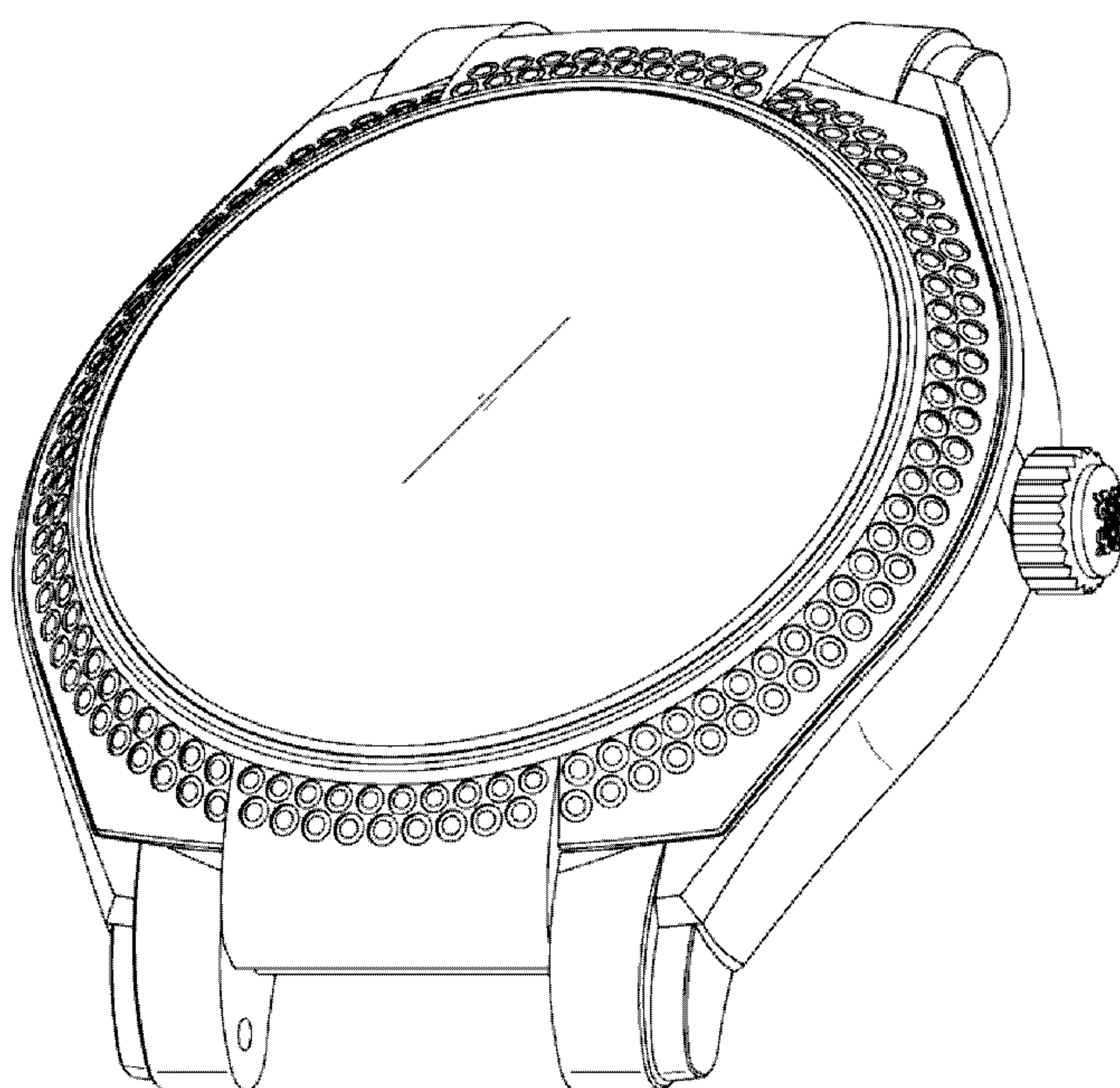
【立體圖】
