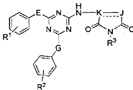
Formule (I)
