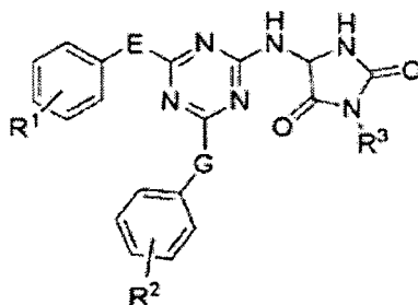
Formule (II)
