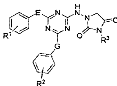
Formule (III)
