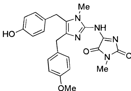
Naamidine A
