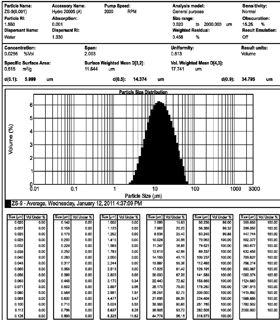
Fig. 4 (ZS-9 preclinical lot)
